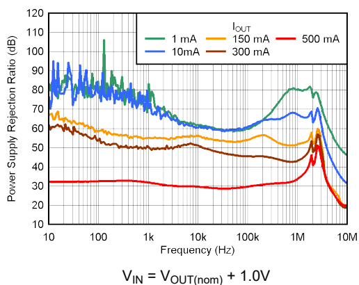
図 5-13. PSRR と周波数との関係
