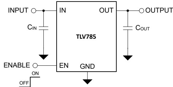
図 7-1. TLV785 の代表的なアプリケーション
