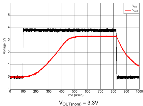
図 5-14. スタートアップ
