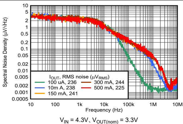
図 5-15. ノイズ
