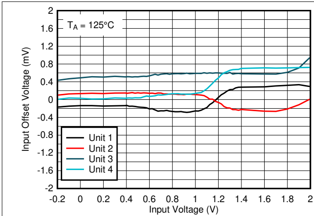
図 5-23. オフセット電圧と入力電圧の関係 (125°C、1.8V)
