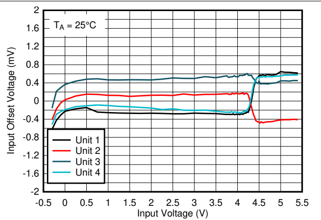
図 5-26. オフセット電圧と入力電圧の関係 (25°C、5V)
