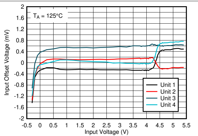
図 5-24. オフセット電圧と入力電圧の関係 (125°C、5V)
