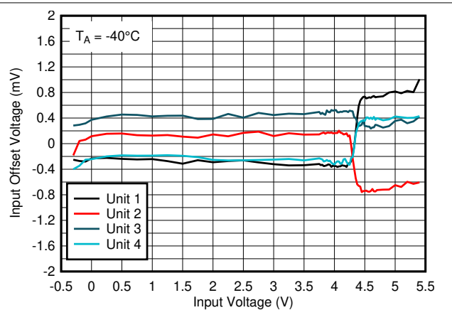
図 5-28. オフセット電圧と入力電圧の関係 (-40°C、5V)
