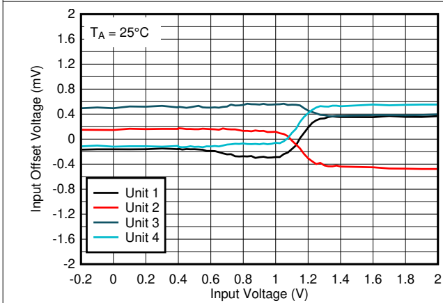
図 5-25. オフセット電圧と入力電圧の関係 (25°C、1.8V)
