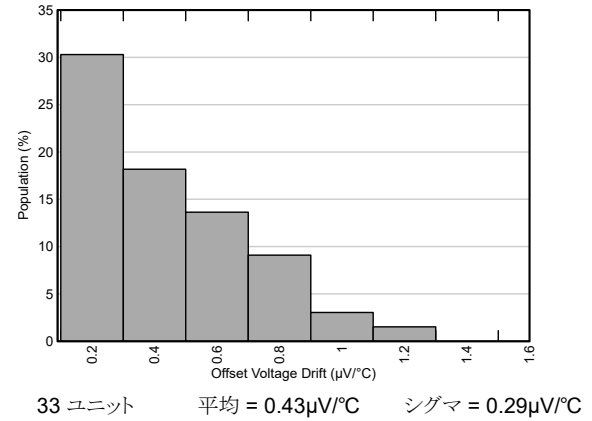
図 5-2. オフセット電圧ドリフトの分布ヒストグラム
