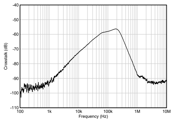
図 5-35. チャネル セパレーション
