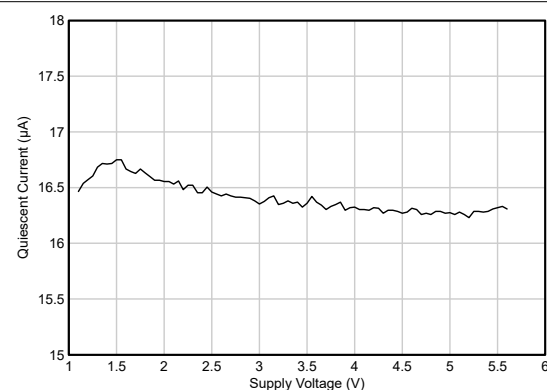
図 5-24. 静止電流と電源電圧との関係
