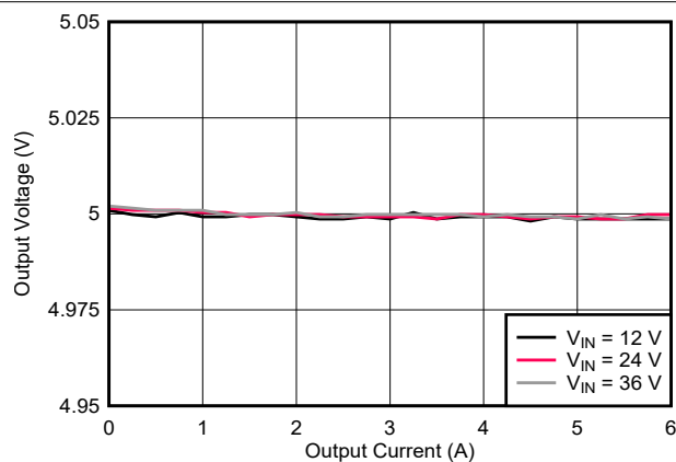
图 9-3. Load Regulation
