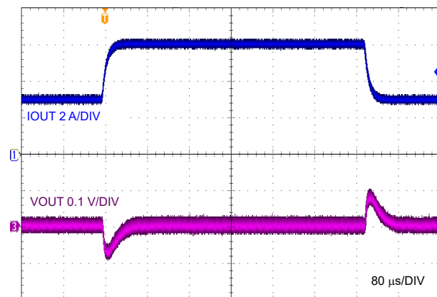
图 9-6. Load Transient, 3 A to 6 A, 1 A/ \mu\text{s}
