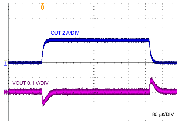
图 9-7. Load Transient, 0 A to 3 A, 1 A/ \mu\text{s}
