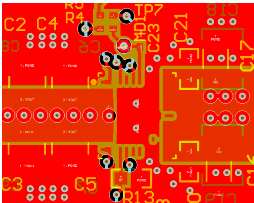
図 7-19. レイアウト例
