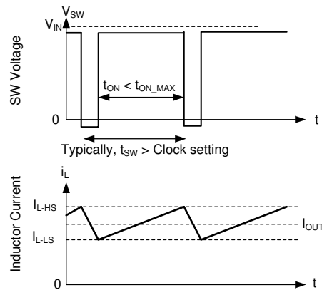
図 6-8. 電流制限波形
