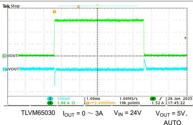
図 7-7. 負荷過渡 (0% ~ 100%)
