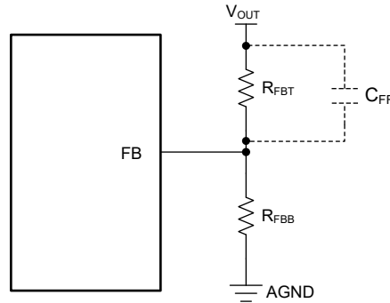
図 6-1. 可変バージョンの出力電圧の設定
