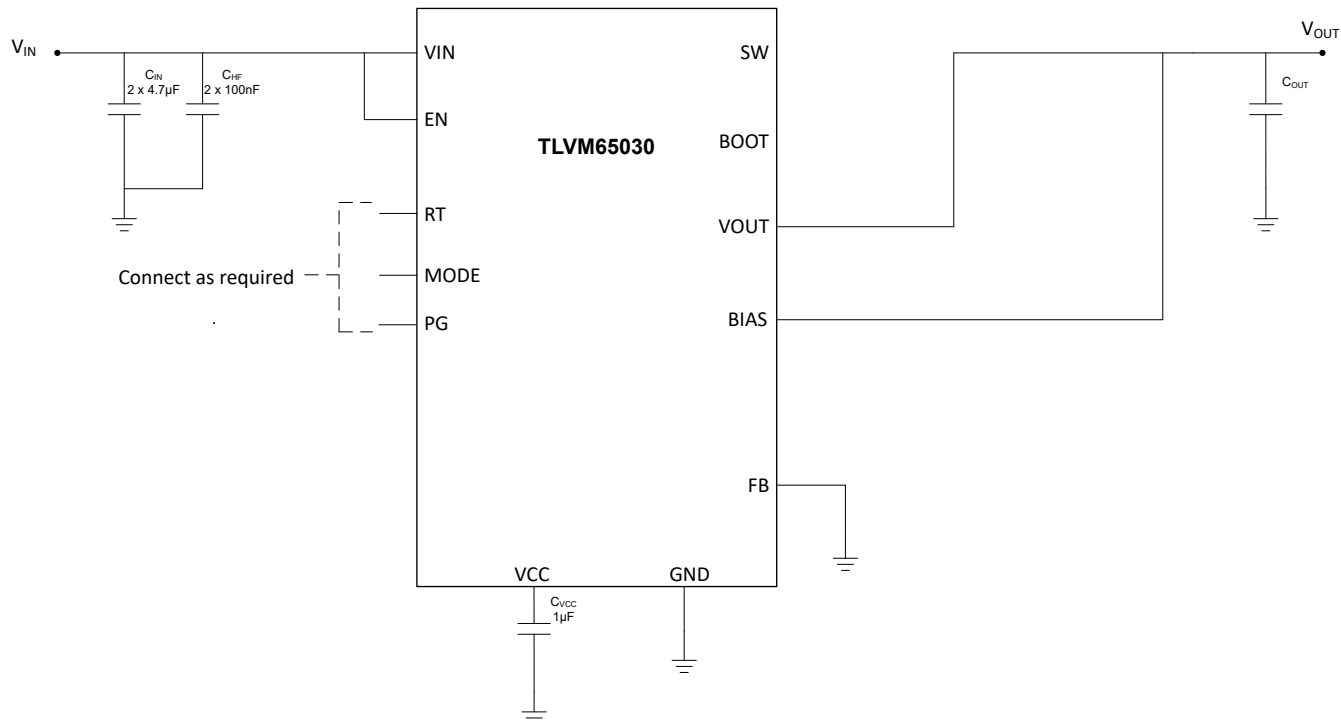
図 7-1. TLVM65030 を用いた固定出力電圧モードのアプリケーション回路例
