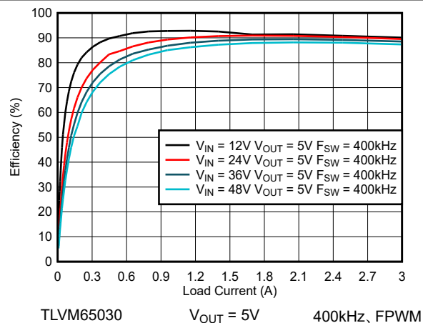
図 7-10. 効率
