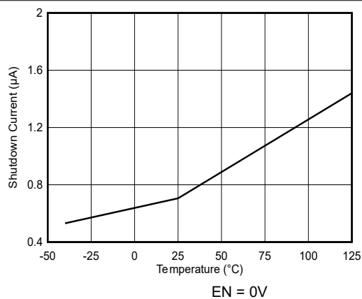
図 5-2. シャットダウン入力電流
