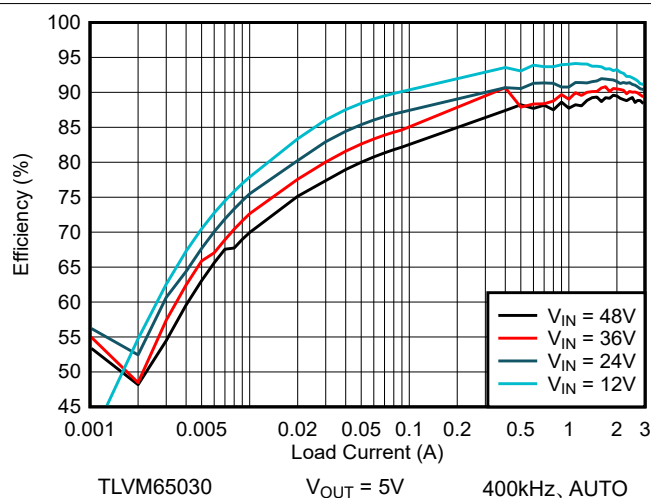
図 7-4. 効率
