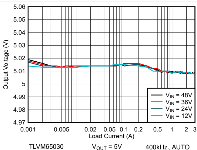
図 7-5. ラインおよびロードレギュレーション
