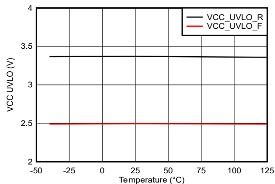
図 5-4. V_{CC} UVLO
