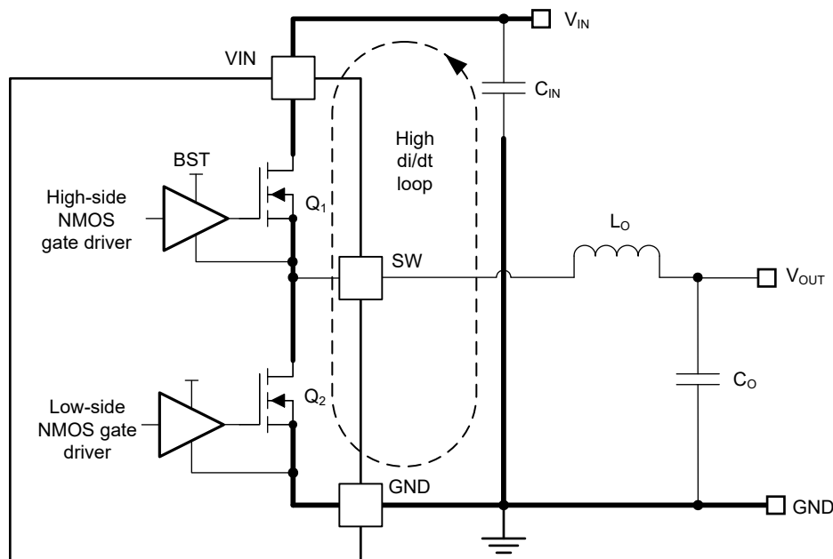
図 7-18. 高速エッジを持つ電流ループ
