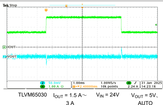
図 7-6. 負荷過渡 (50% ~ 100%)
