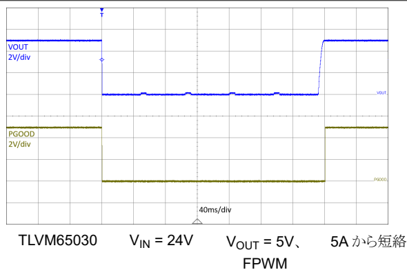
図 7-12. 短絡発生
