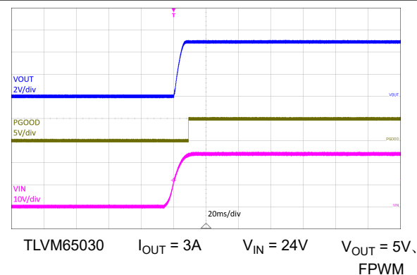
図 7-15. スタートアップ
