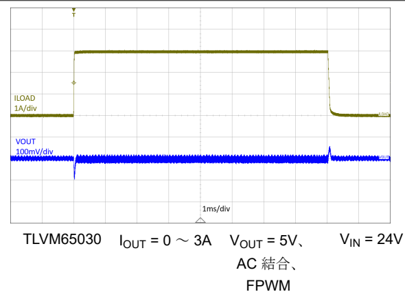
図 7-13. 負荷過渡 (0 ~ 100%)
