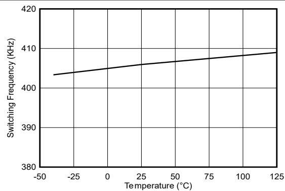
図 5-6. f_{SW} 400kHz
