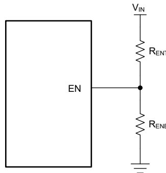
図 6-2. EN ピンを使った VIN/UVLO
