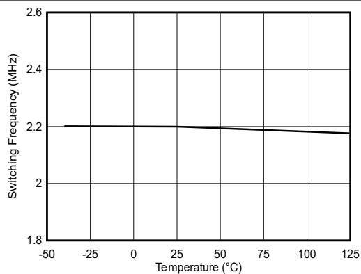
図 5-5. f_{SW} 2.2MHz
