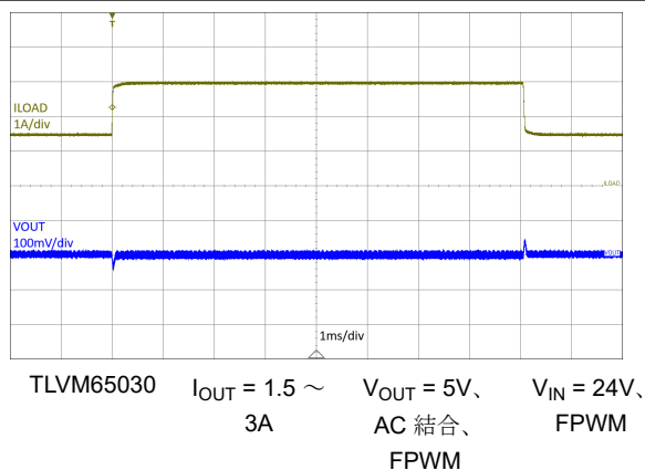
図 7-14. 負荷過渡 (50 ~ 100%)
