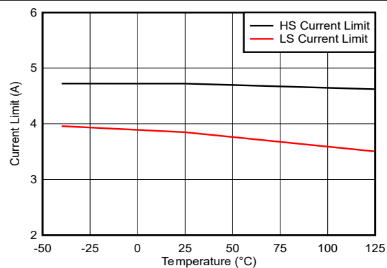
図 5-8. 電流制限
