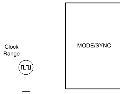
図 6-3. MODE/SYNC ピンを使用した同期ができる代表的な実装
