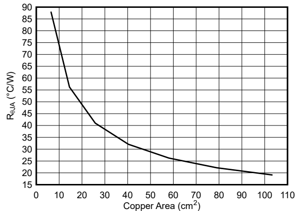
図 7-3. 熱抵抗と銅面積との関係
