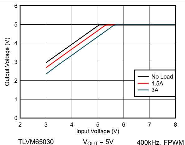
図 7-11. ドロップアウト
