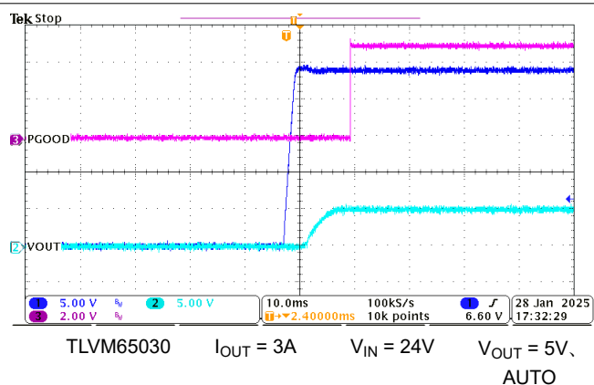
図 7-8. スタートアップ
