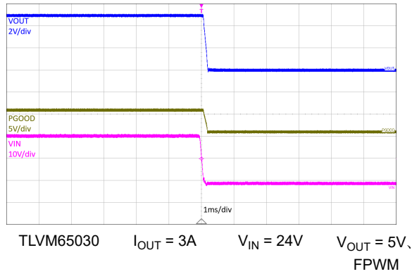
図 7-16. シャットダウン
