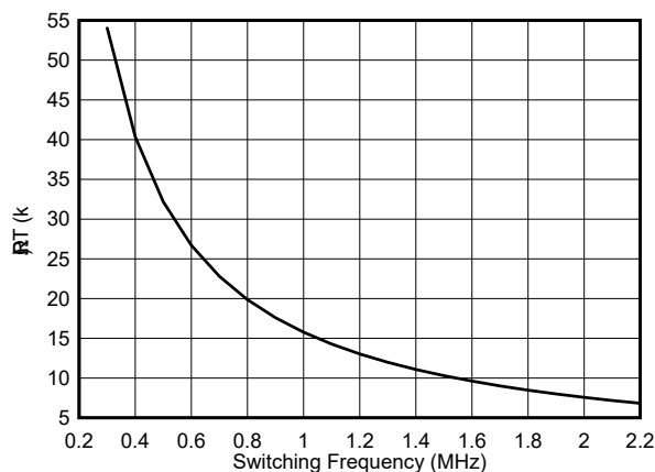
図 6-6. スwitchング周波数と RT との関係
