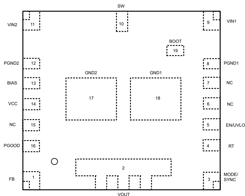
図 4-1. 19 ピン VCG、QFN-FCMOD パッケージ (上面図)
