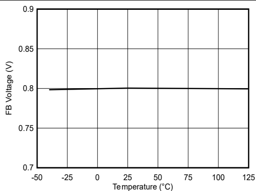
図 5-1. 帰還電圧
