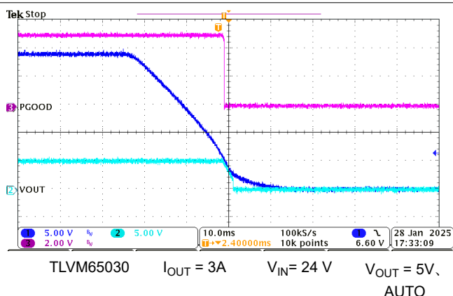
図 7-9. シャットダウン
