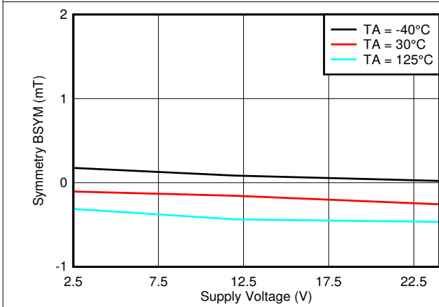
图 7-59. B_{SYM(x)} vs. V_{CC}
