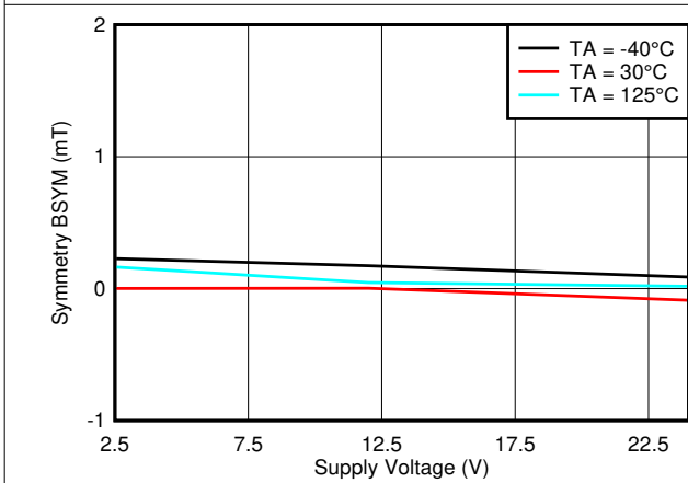
图 7-61. B_{SYM(y)} vs. V_{CC}
