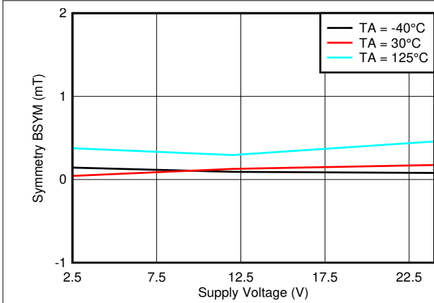
图 7-57. B_{SYM(z)} vs. V_{CC}
