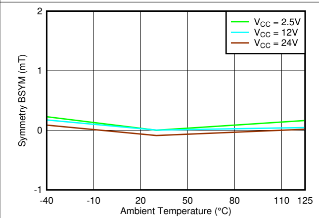
图 7-62. B_{SYM(y)} vs. Temperature
