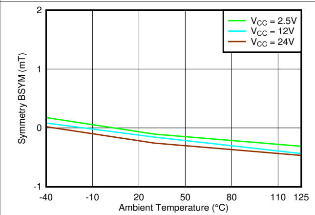
图 7-60. B_{SYM(x)} vs. Temperature
