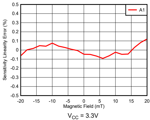
図 6-1. TMAG5253BA1 感度直線性誤差と磁界との関係
