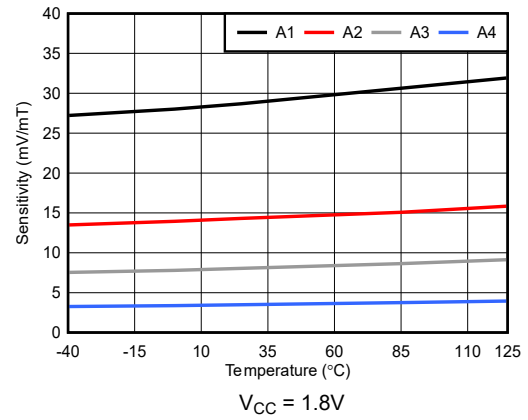
図 6-8. TMAG5253BA 感度と温度との関係 V_{CC} = 1.8\text{V}
