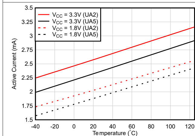
図 6-17. 電源電流と温度との関係
