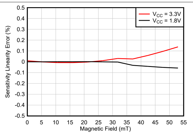
図 6-14. TMAG5253UA5 感度直線性誤差と磁界との関係
