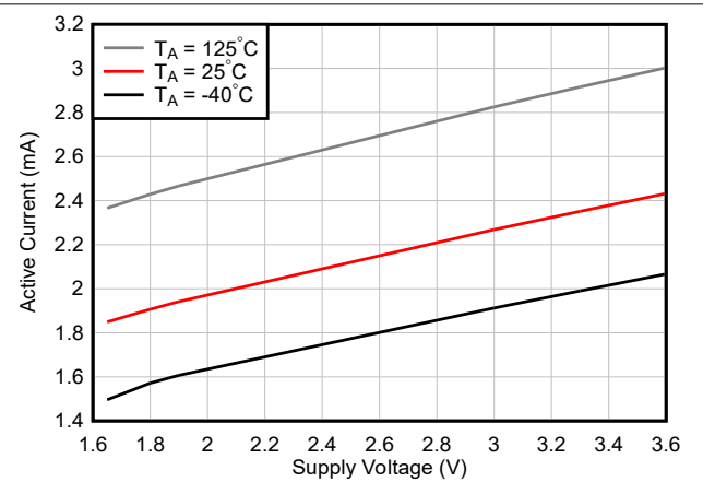
図 6-16. TMAG5253UA5 電源電流と電源電圧との関係
