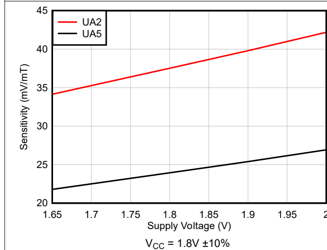
図 6-21. 感度と電源電圧との関係
