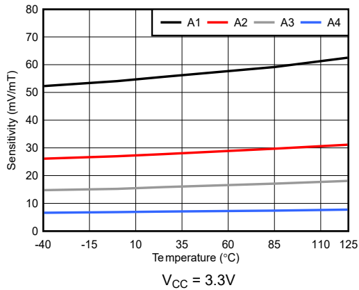
図 6-9. TMAG5253BA 感度と温度との関係 V_{CC} = 3.3\text{V}
