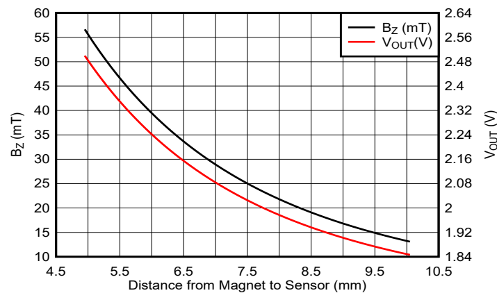
図 9-9. 磁界 (B Z ) およびセンサの出力電圧 (V OUT ) と磁石から TMAG5253B でのセンサまでの距離との関係
