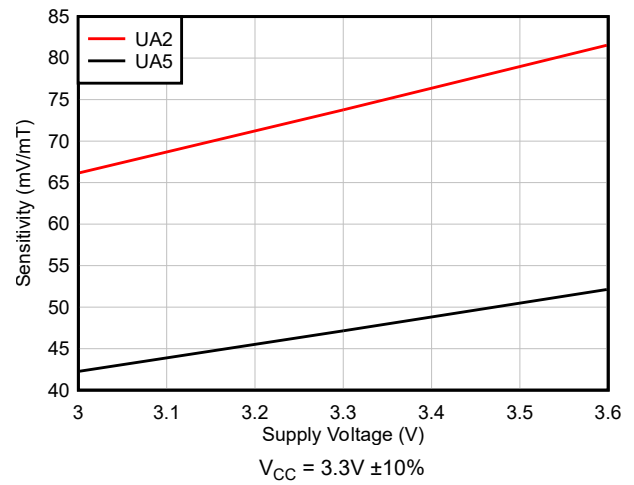
図 6-20. 感度と電源電圧との関係
