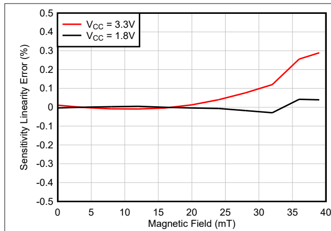
図 6-13. TMAG5253UA2 感度直線性誤差と磁界との関係
