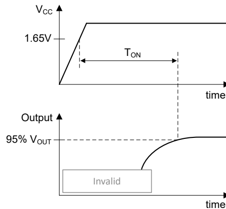
図 7-5. V_{CC} ランプの T_{ON}
