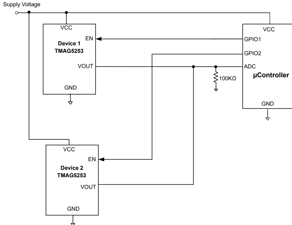
図 9-1. 共有出力を持つ複数のセンサ
