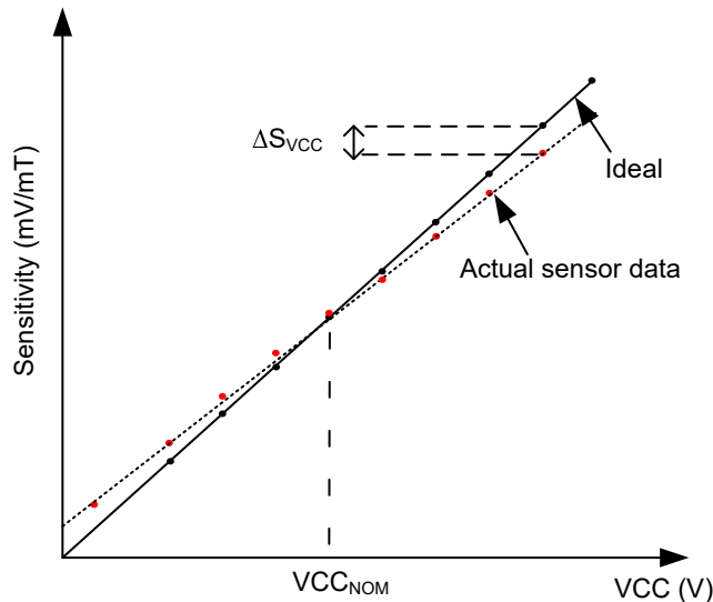
図 7-3. 感度のレシオメトリック誤差
