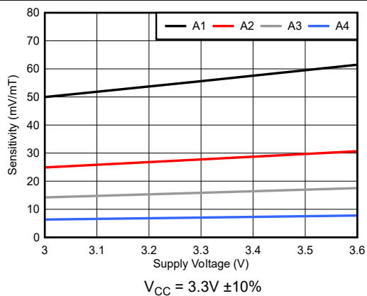
図 6-11. TMAG5253BA 感度と電源電圧との関係 V_{CC} = 3.3\text{V} \pm 10\%
