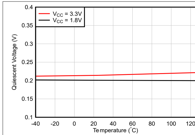
図 6-19. TMAG5253UA 静止電圧と温度との関係
