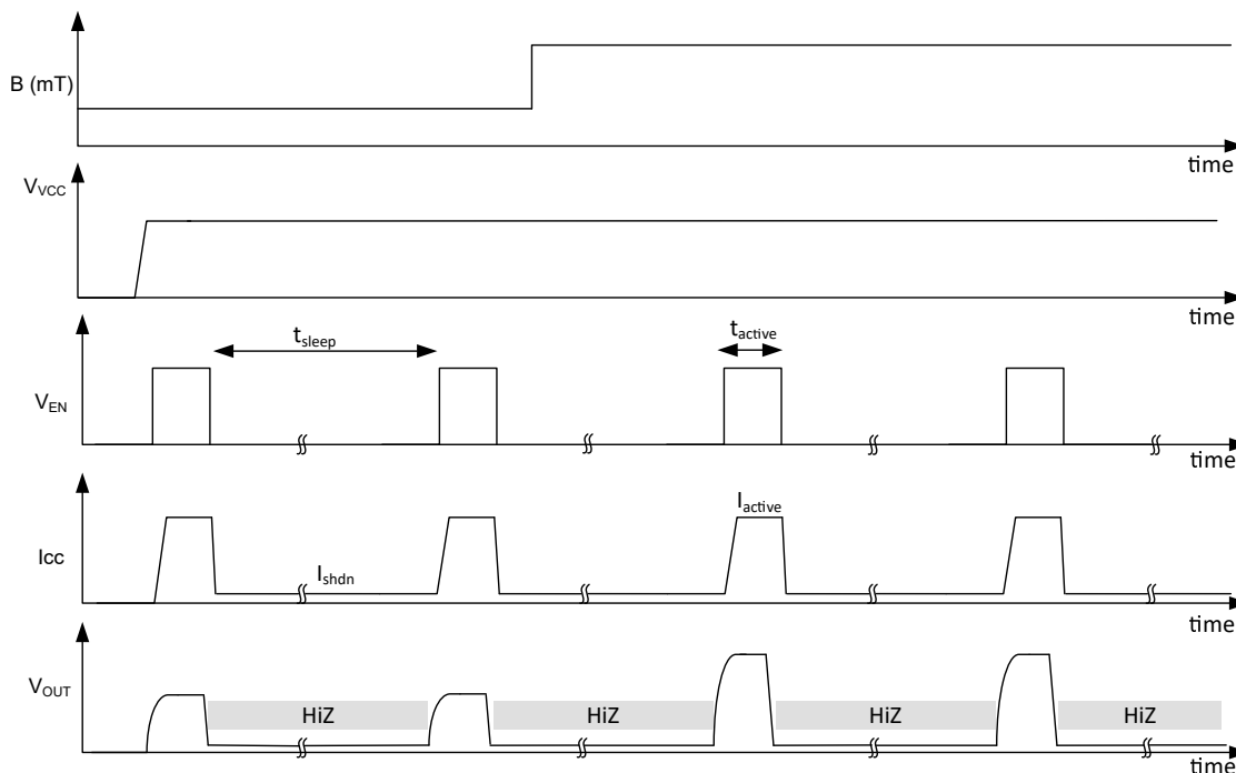
図 9-4. デューティ サイクル アプリケーションのタイミング図
