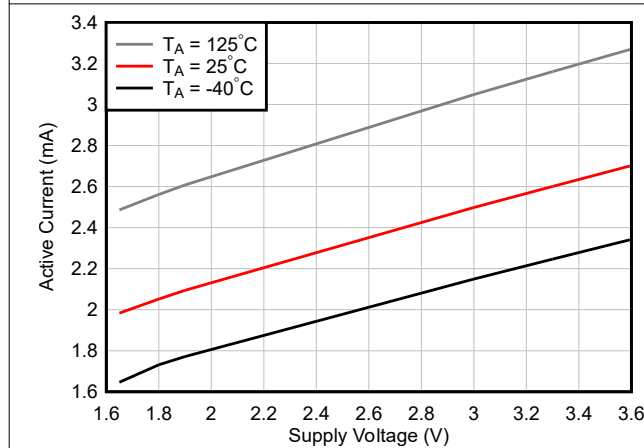
図 6-15. TMAG5253UA2 電源電流と電源電圧との関係
