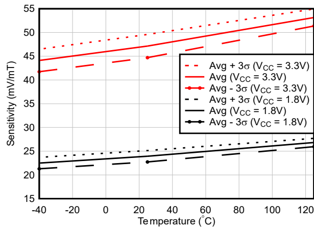
図 6-23. TMAG5253UA5 感度と温度との関係
