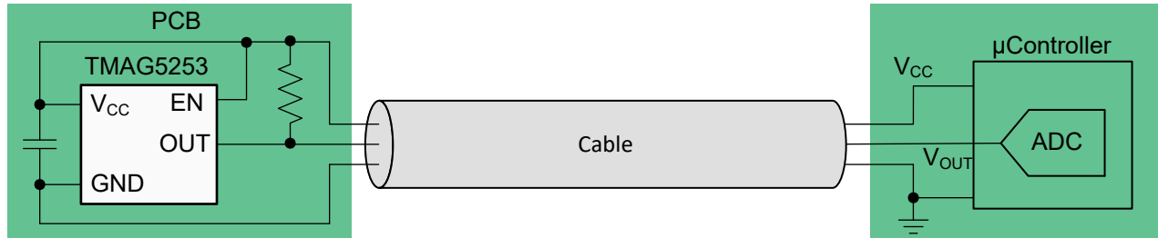
図 9-10. ワイヤ破損検出機能を備えたリモートセンシング アプリケーション
