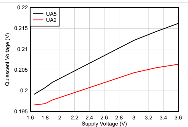
図 6-18. 静止電圧と電源電圧との関係
