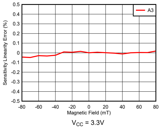
図 6-3. TMAG5253BA3 感度直線性誤差と磁界との関係
