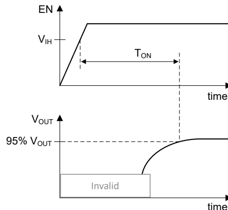
図 7-6. EN ピン使用時の T_{ON}
