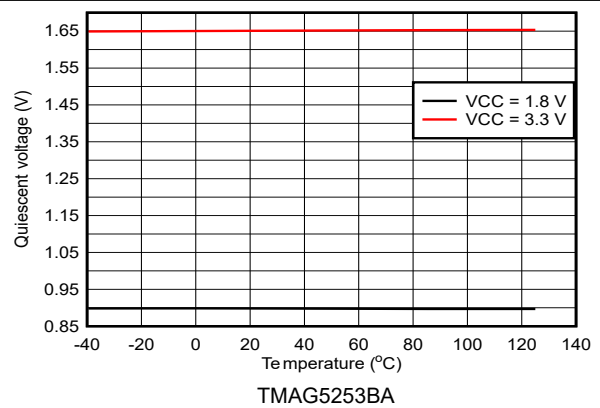
図 6-12. TMAG5253BA 静止電圧と温度との関係
