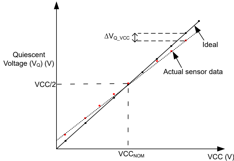
図 7-4. 静止のレシオメトリック誤差
