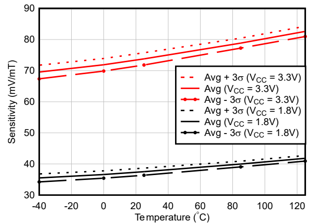
図 6-22. TMAG5253UA2 感度と温度との関係
