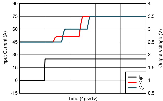
図 8-12. 1V の出力スイングに十分な入力電流ステップに対する過渡応答
