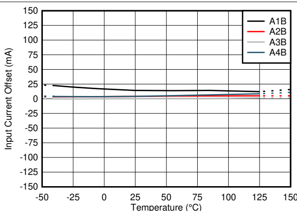
図 6-3. TMCS1101AxB の入力オフセット電流と温度との関係
