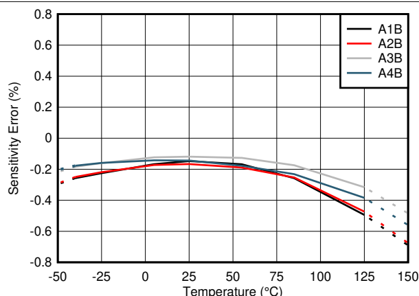
図 6-1. TMCS1101AxB の感度誤差と温度との関係
