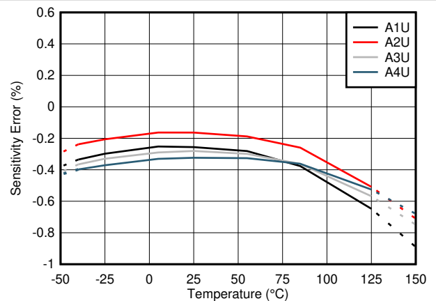
図 8-5. 温度範囲全体での感度ドリフト (U バリエーション)
