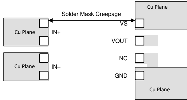
図 9-4. システムの沿面距離要件を満たすレイアウト
