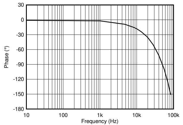
図 6-18. 位相と周波数との関係、すべてのゲイン
