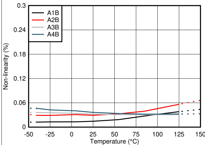
図 6-5. 非線形性線性と温度との関係
