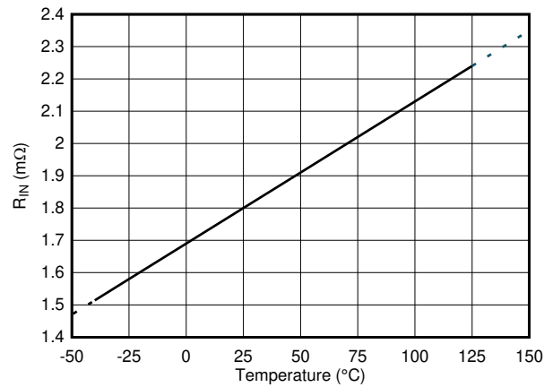
図 6-27. 入力導体の抵抗と温度との関係
