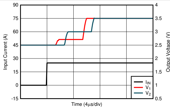
図 6-23. 電圧出カステップ、立ち上がり
