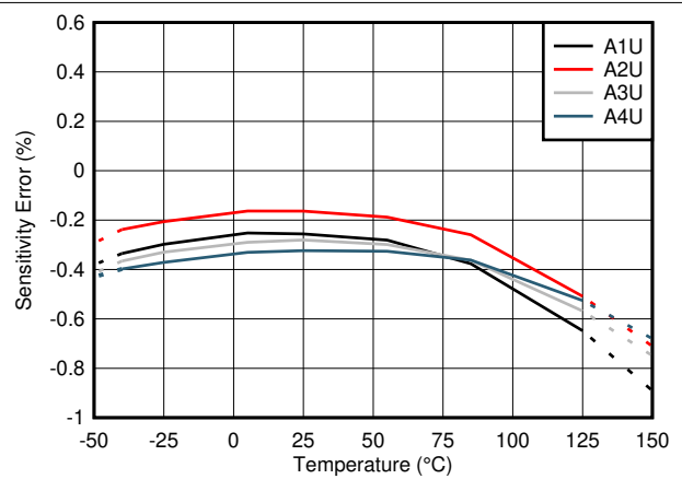
図 6-2. TMCS1101AxU の感度誤差と温度との関係
