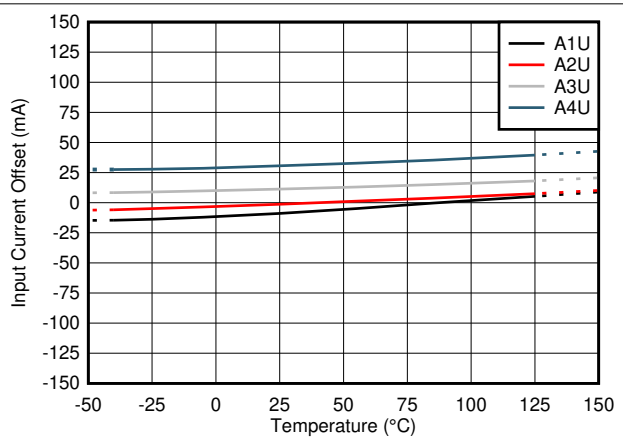
図 6-4. TMCS1101AxU の入力オフセット電流と温度との関係
