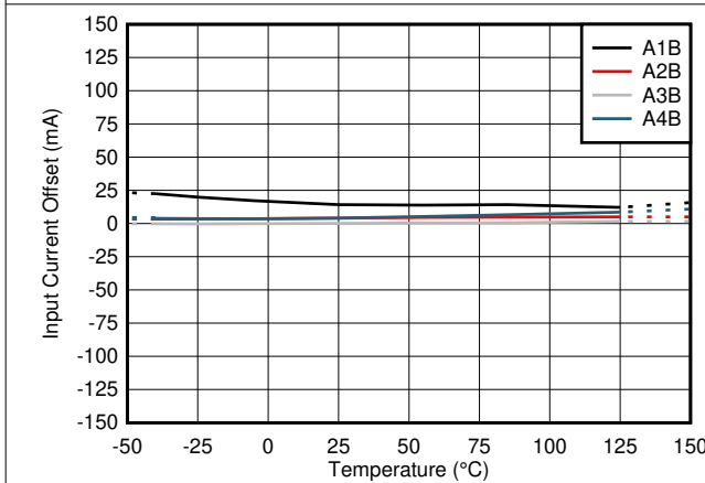
図 6-3. TMCS1101AxB の入力オフセット電流と温度との関係
