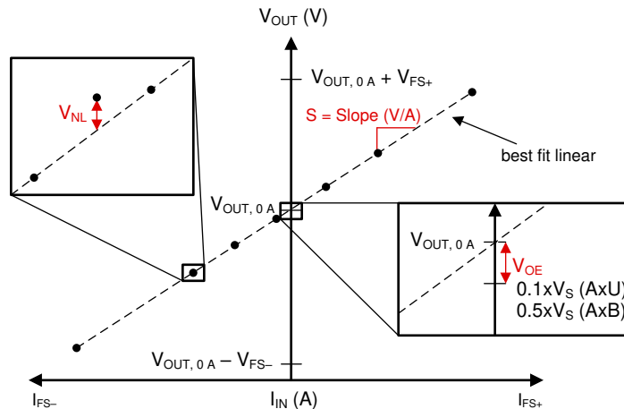
図 7-1. 感度、オフセット、非直線性誤差
