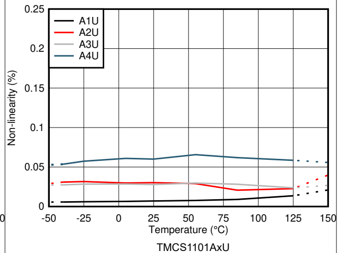
図 6-6. 非線形性線性と温度との関係
