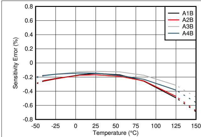
図 6-1. TMCS1101AxB の感度誤差と温度との関係
