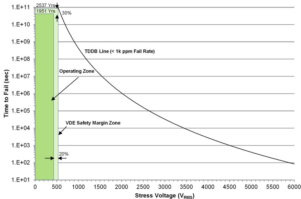
図 8-1. 絶縁寿命
