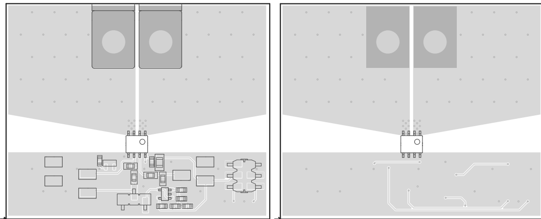
図 9-5. 基板の上面 (左) と底面 (右) プレーンの推奨レイアウト
