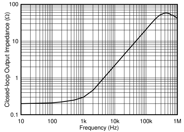
図 6-20. 出カインピーダンス 対 周波数
