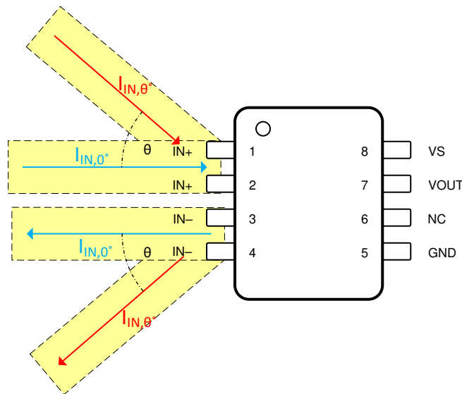
図 9-3. 入力電流の配線によって発生する磁界
