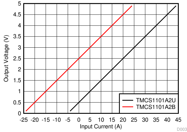
図 8-14. TMCS1101A2B および TMCS1101A2U の出力電圧と入力電流の関係
