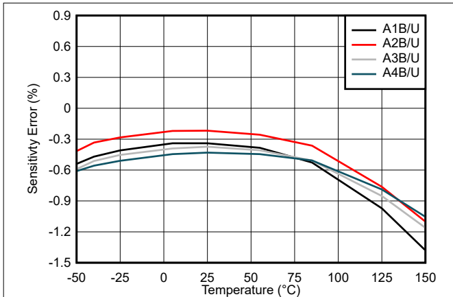
図 7-1. TMCS1108 感度誤差と温度との関係
