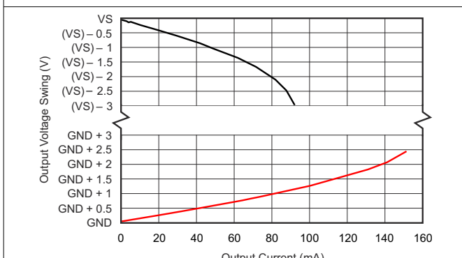
図 7-5. 出力電圧スイングと出力電流との関係
