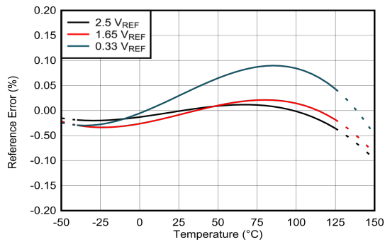
図 6-3. 基準誤差と温度との関係
