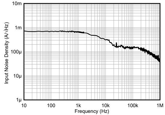
図 6-22. 入力換算ノイズ密度と周波数との関係
