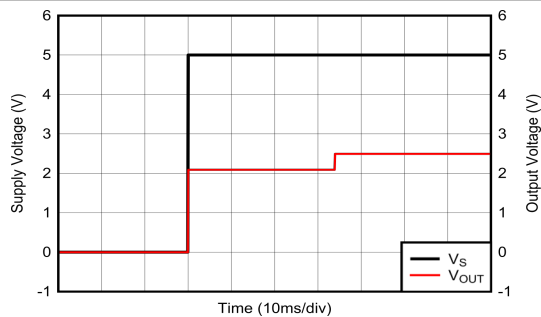
図 6-19. スタートアップ過渡応答
