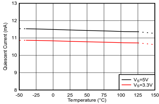
図 6-21. 静止電流と温度との関係
