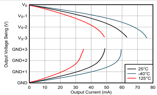
図 6-20. 出力スイングと出力電流との関係
