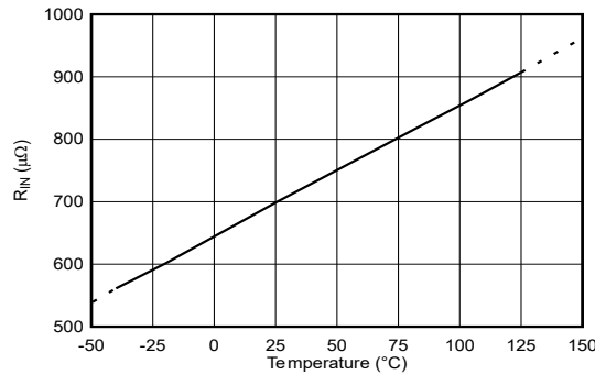
図 6-23. 入力導体の抵抗と温度との関係
