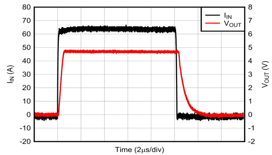
図 6-18. 過電流パラメータ
