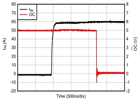
図 6-17. マスクによる過電流出力応答
