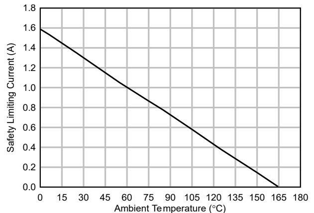
図 6-25. 安全性制限電流による熱特性低下曲線、サイド 2
