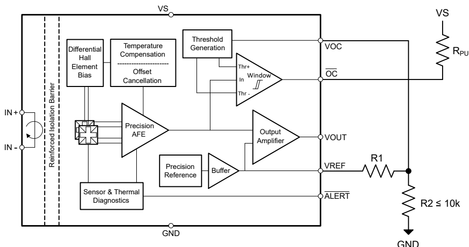
図 8-7. ゼロ電流出力基準電圧を使用するユーザーが構成可能な過電流スレッシュホールド
