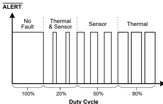
図 8-10. センサ診断波形
