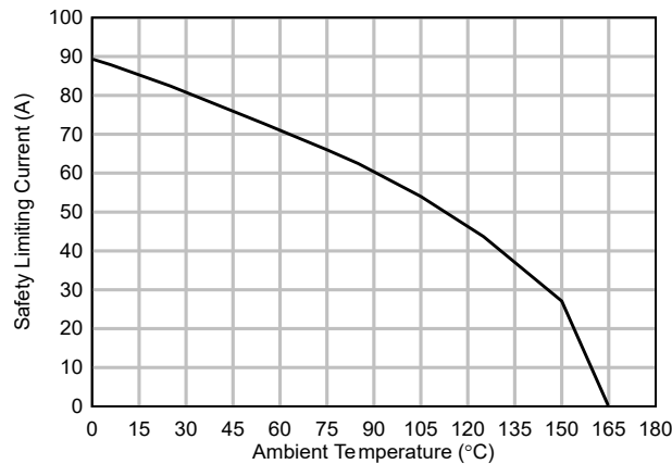
図 6-24. 安全性制限電流による熱特性低下曲線、サイド 1
