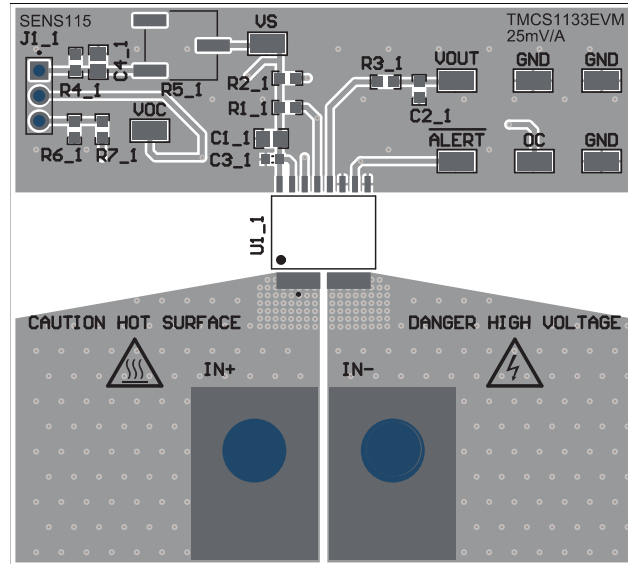
図 9-6. 推奨されるボードレイアウト
