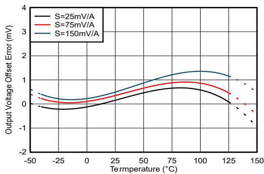
図 6-3. オフセット誤差と温度との関係： TMCS1133Bxx-Q1 のデバイスオプション
