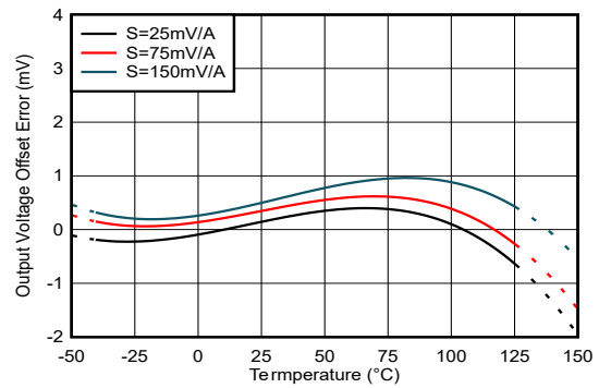
図 6-2. オフセット誤差と温度との関係： TMCS1133Axx-Q1 のデバイス オプション
