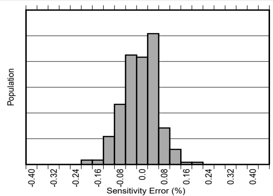
すべての感度 図 6-6. 感度誤差の製品分布
