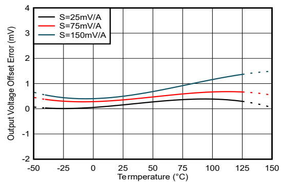
図 6-4. オフセット誤差と温度との関係： TMCS1133Cxx-Q1 のデバイスオプション
