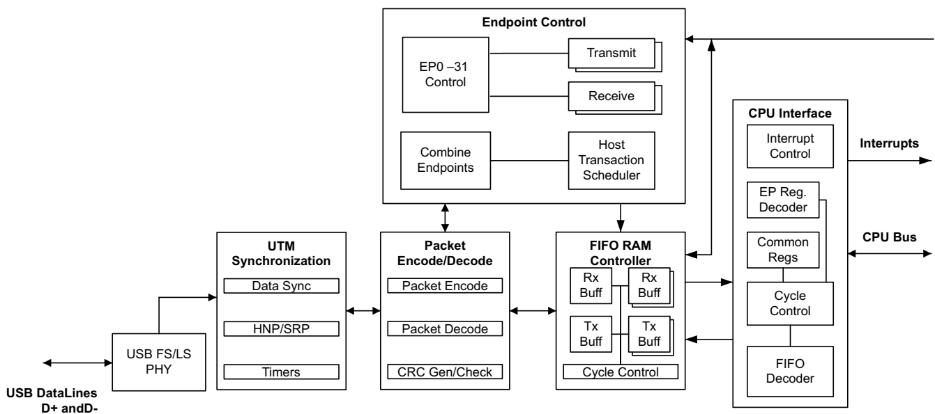
図 6-77. USB ブロック図
