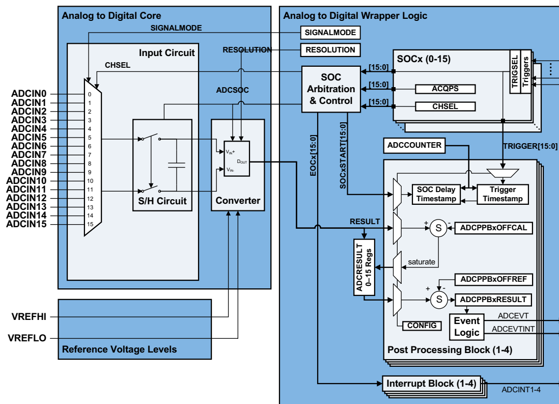
図 6-33. ADC モジュールのブロック図
