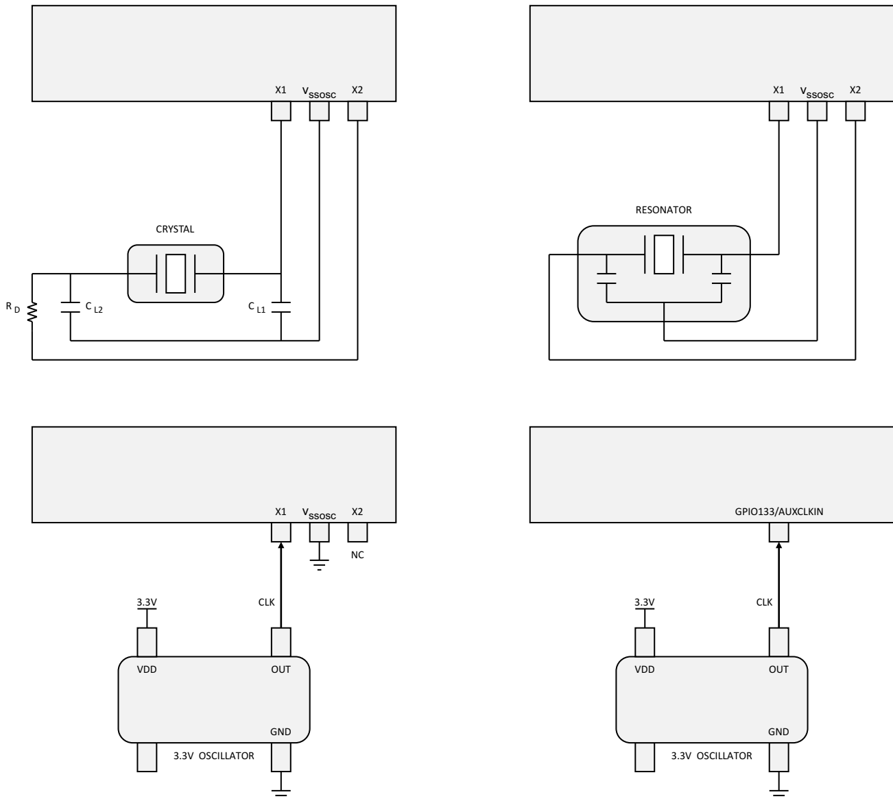
図 6-8. 2807x デバイスへの入カクロックの接続
