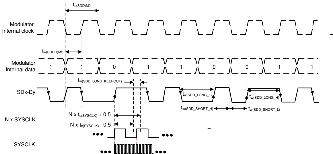
図 6-59. SDFM タイミング図 - モード 2
