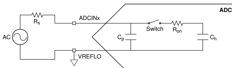
図 6-35. シングルエンド入力モデル
