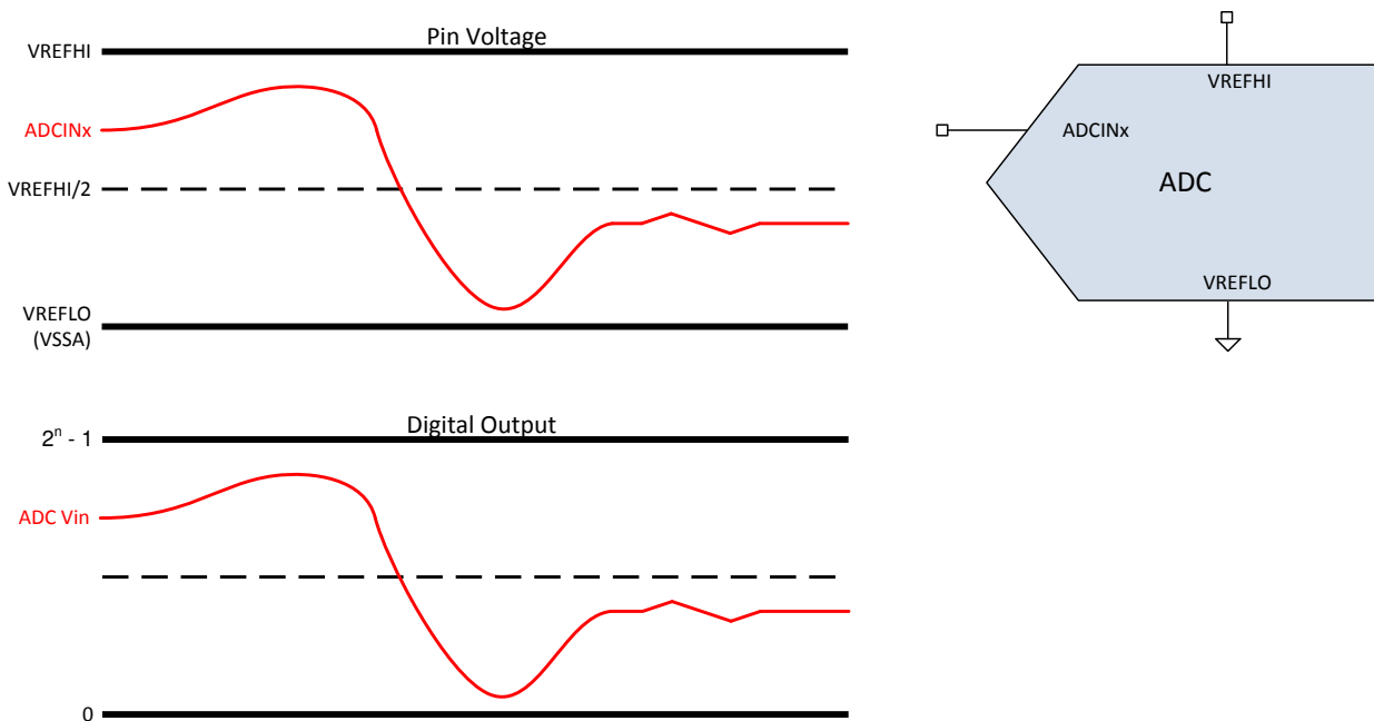
図 6-34. シングルエンド信号モード
