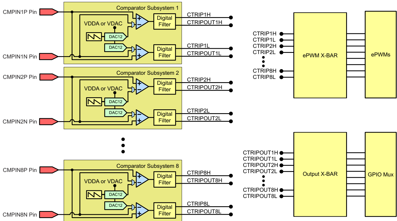
図 6-37. CMPSS 接続 (176 ピン PTP)
