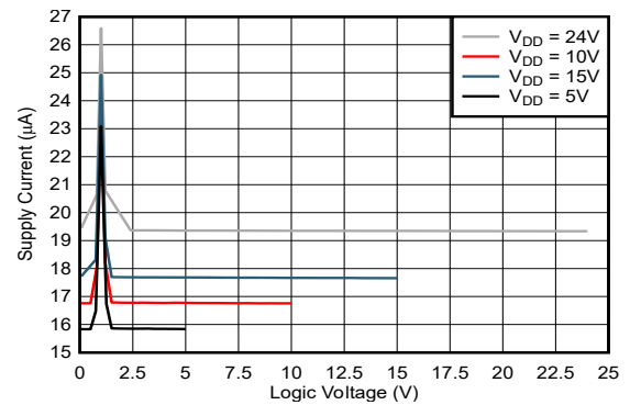
図 5-4. 電源電流とロジック電圧との関係
