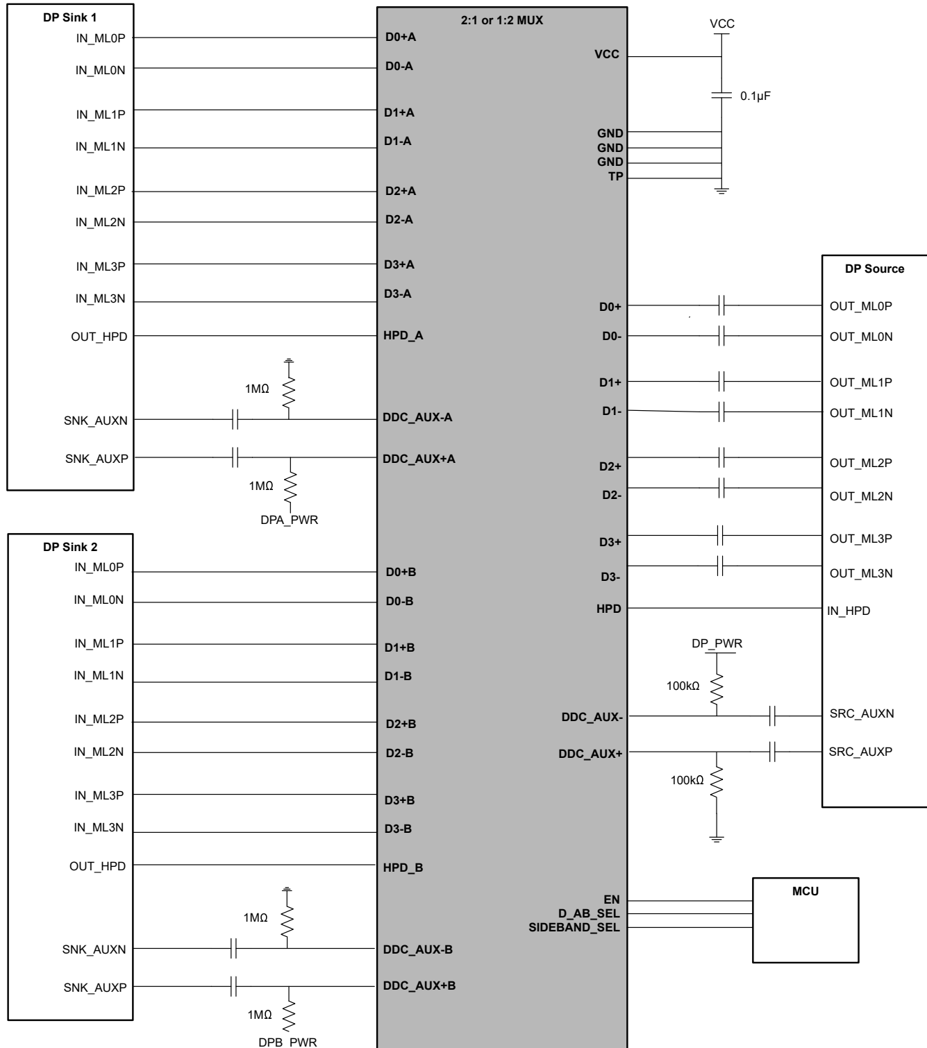
8-8. DisplayPort 1:2 Switching
