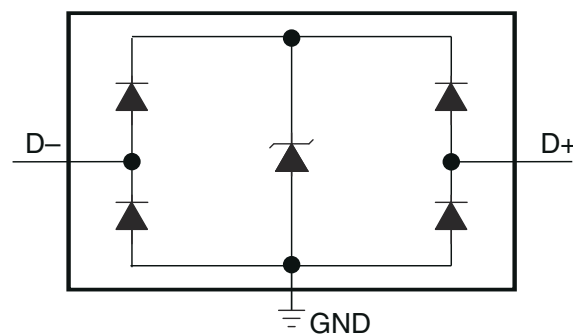
TPD2EUSB30/A の回路図
