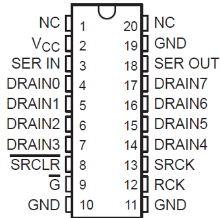
図 4-1. DW または N パッケージ（上面図）
