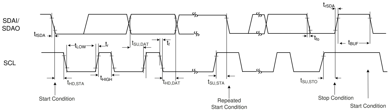
图 31. I 2 C Timings
