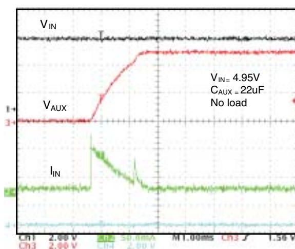
イネーブル後のブースト・スタートアップ - 無負荷
