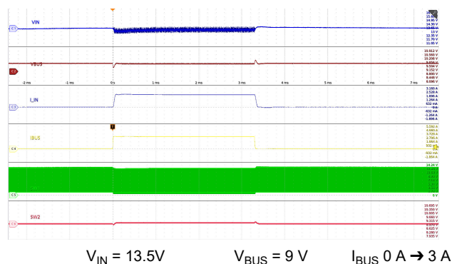
図 9-31. Load Transient (Buck): V_{BUS} = 9\text{ V}
