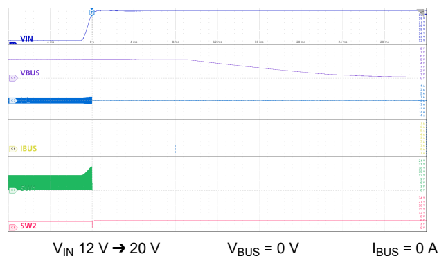
図 9-29. V_{IN(OVP)} Showing V_{BUS} Discharge
