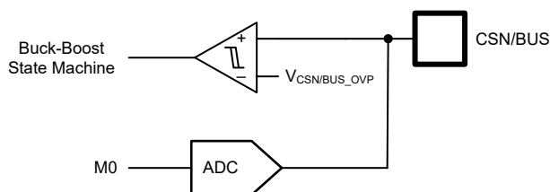
図 8-18. V_{BUS} OVP and UVP
