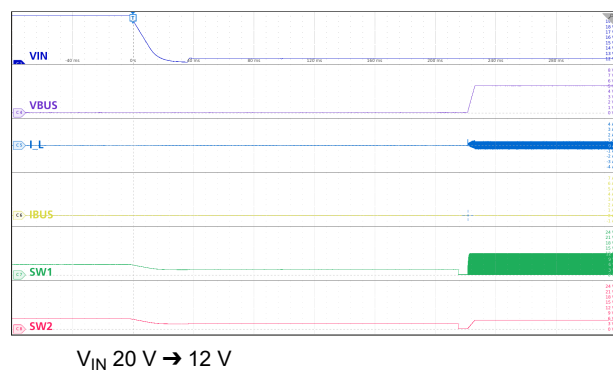
図 9-28. V_{IN(OVP)} Recovery
