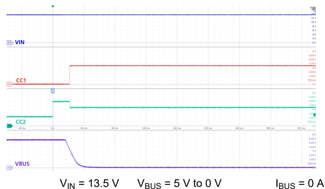
図 9-13. Type-C Detach
