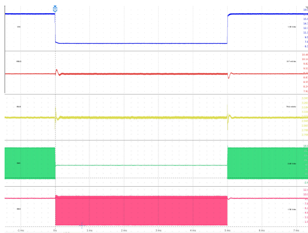
図 9-35. Line Transient: V_{BUS} = 20V
