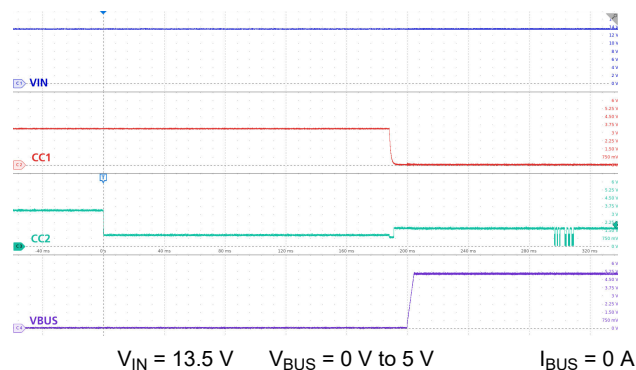
図 9-12. Type-C Attach
