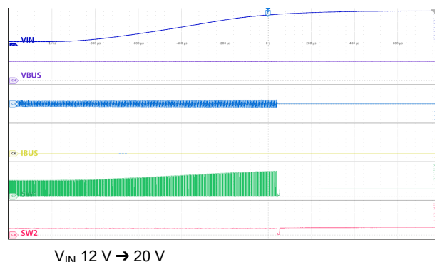
図 9-27. V_{IN(OVP)} Entry
