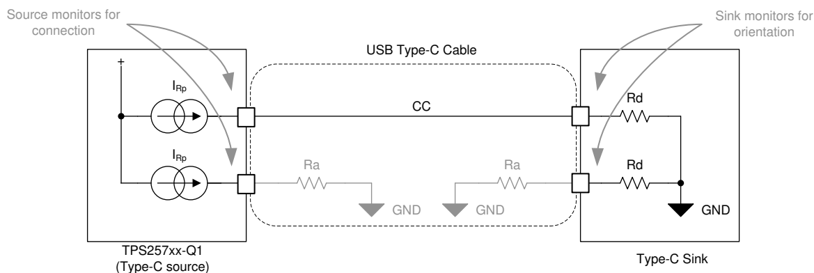
図 8-29. Type-C Cable
