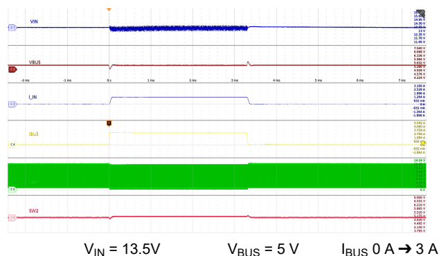
図 9-30. Load Transient (Buck): V_{BUS} = 5\text{ V}
