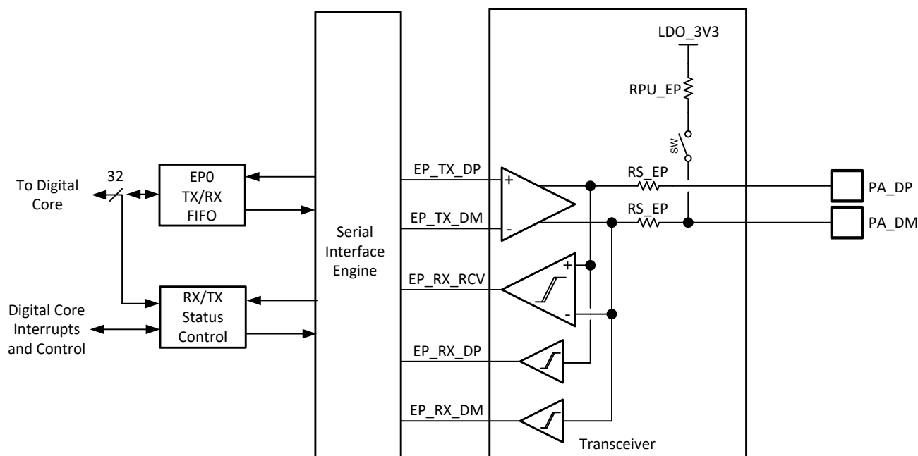
図 8-34. USB Endpoint PHY
