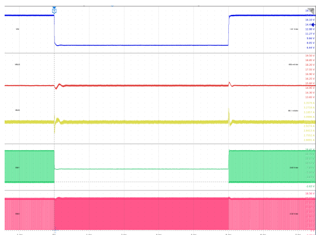
図 9-36. Line Transient: V_{BUS} = 15V
