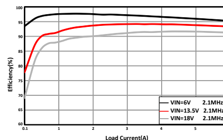
効率と出力電流との関係
