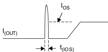
FIG 9-5. Output Short-Circuit Parameters
