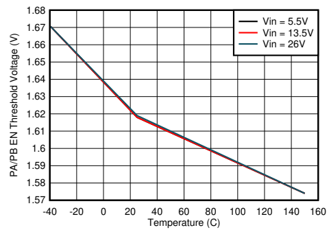
8-4. Precision USB PA/PB Enable Threshold
