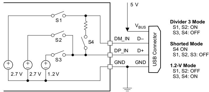
10-24. DCP Auto Mode
