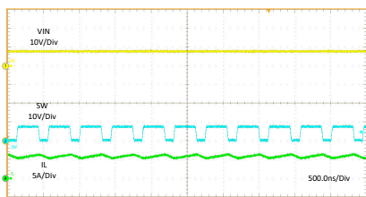
VIN = 8 V L = 0.68 \mu H I PA_BUS = 3 A I PB_BUS = 3 A
