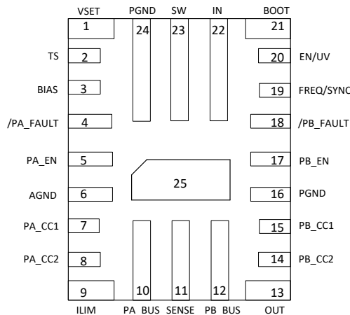
7-3. TPS25852-Q1 RPQ Package 25-Pin (QFN) Top View
