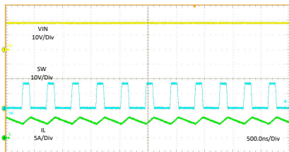
VIN = 18 V L = 0.68 \mu H I PA_BUS = 3 A I PB_BUS = 3 A
