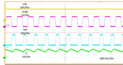
VIN = 18 V L = 0.68 \mu H I PA_BUS = 3 A I PB_BUS = 3 A
