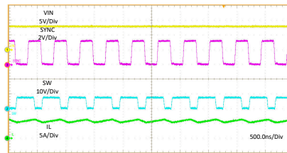
VIN = 8 V L = 0.68 \mu H I PA_BUS = 3 A I PB_BUS = 3 A
