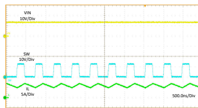
VIN = 13.5 V L = 0.68 \mu H I PA_BUS = 3 A I PB_BUS = 3 A
