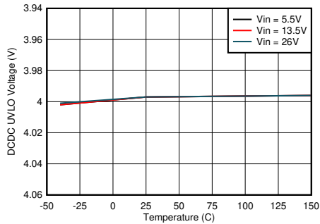
8-7. DCDC UVLO Threshold
