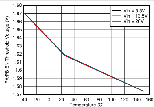
FIG 8-4. Precision USB PA/PB Enable Threshold
