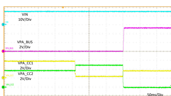
11-18. Startup Relate to EN
