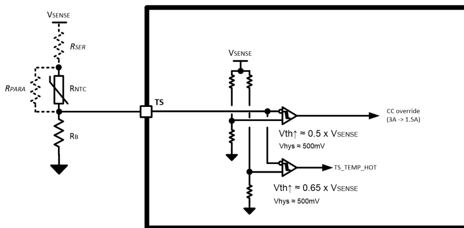
10-10. TS Input
