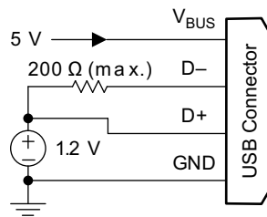
10-18. 1.2-V Mode
