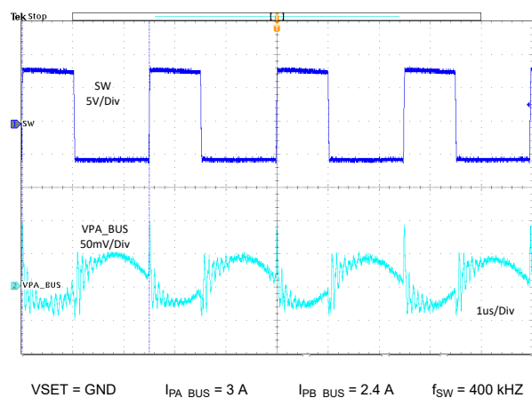
11-13. 6-A Output Ripple
