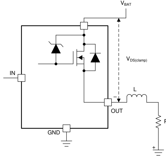
図 8-24. ドレイン-ソース間クランプ構造
