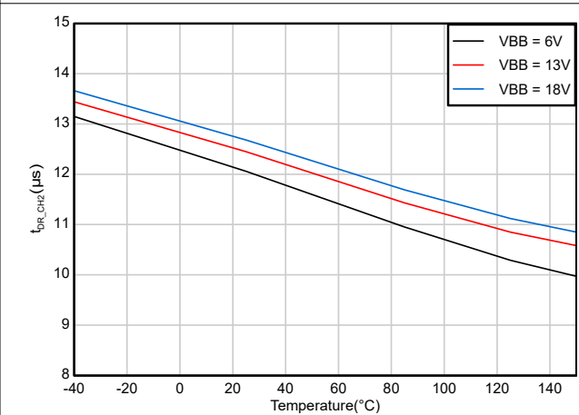
図 6-10. チャネル ターンオン遅延時間 ( t_{DR\_CH2} ) 対 温度 (チャネル 2)
