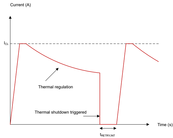
図 8-14. サーマル レギュレーションによる短絡へのイネーブル
