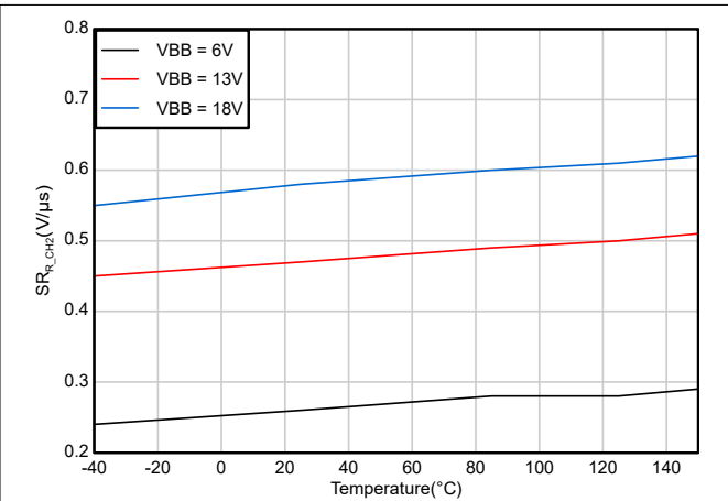
図 6-14. VOUT 上昇スルー レート (SR R ) 対 温度 (チャンネル 2 : P パッケージ)
