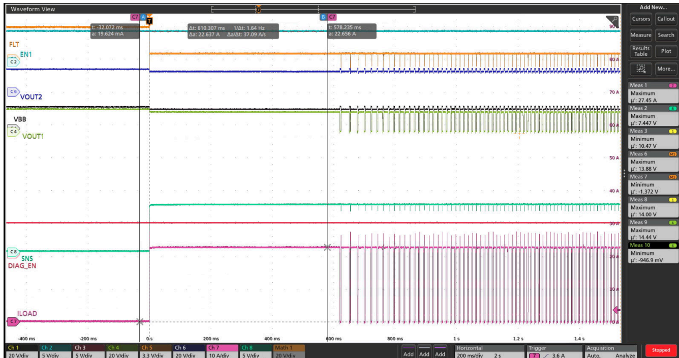
図 8-19. 電流制限 (ILIM=GND) 未滿の負荷電流 (22A 電子負荷) における無限サーマル シャットダウンの再試行動作
