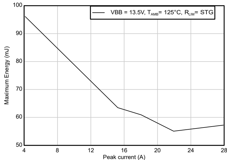
図 8-29. 誘導性スイッチ オフ時の最大エネルギー吸収量 対 ピーク電流 (シングルパルス、VBB = 13.5V、TA = 125°C)
