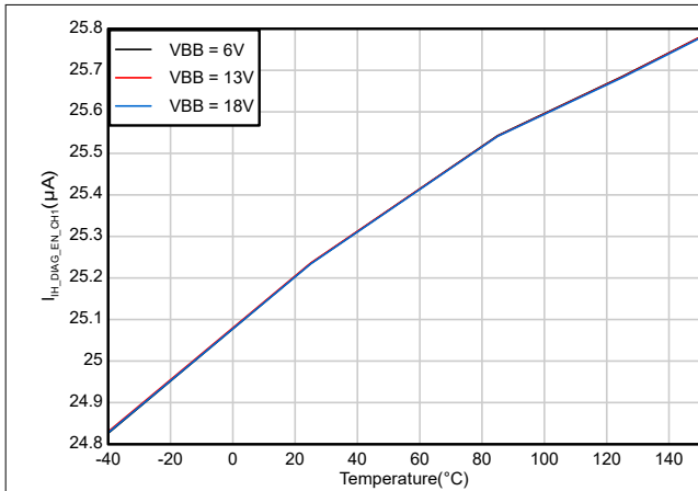
図 6-25. DIAG_EN 入力 電流 高レベル 対 温度
