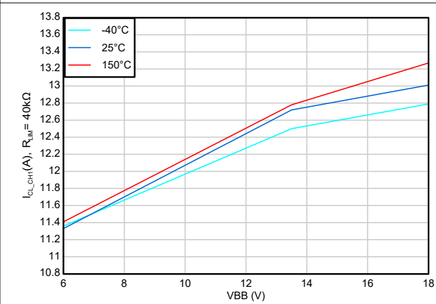
図 6-30. 電流制限レギュレーションレベル (I CL ) 対 VBB (チャネル 1)、R LIM = 40kΩ
