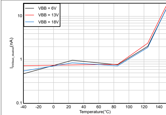
図 6-7. I_{SNS} リーク電流 (Diagnostics 無効時) 対 温度
