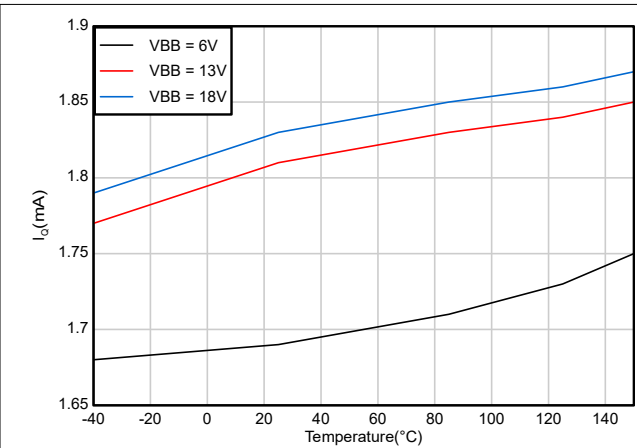
図 6-2. 静止電流 ( I_Q ) 対温度特性 (両チャンネル有効時)
