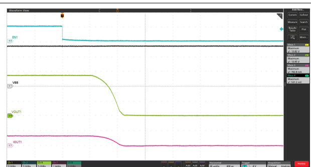
図 9-4. 抵抗性負荷でのターンオフ
