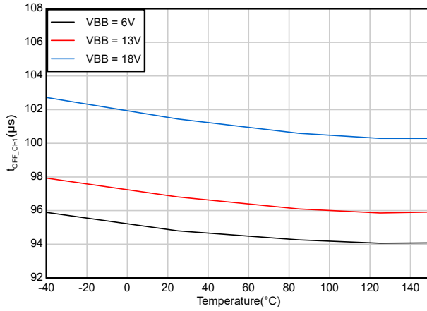
図 6-19. チャンネル ターンオフ時間 ( t_{OFF} ) 対 温度 (チャンネル 1)
