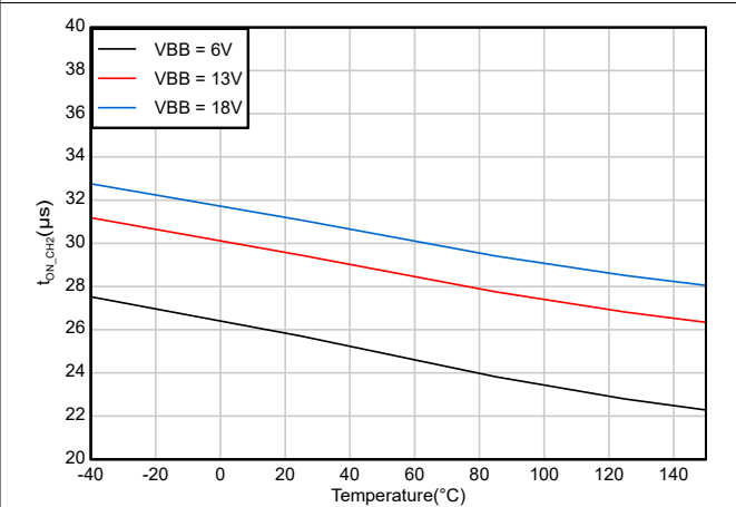
図 6-18. チャンネル ターンオン時間 (t ON ) 対 温度 (チャンネル 2)
