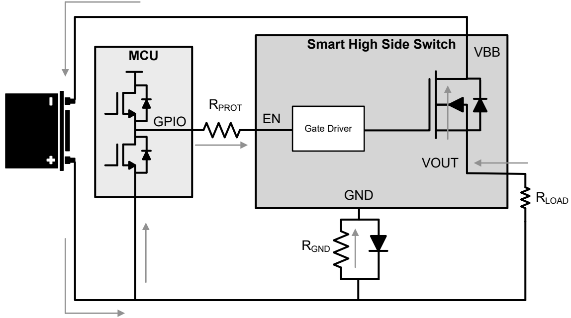
図 8-39. 逆バッテリー回路
