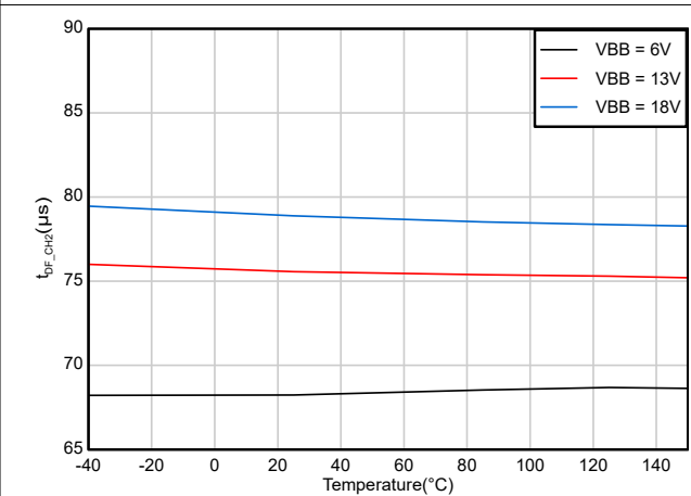
図 6-12. チャネル ターンオフ遅延時間 ( t_{DF} ) 対 温度 (チャネル 2)
