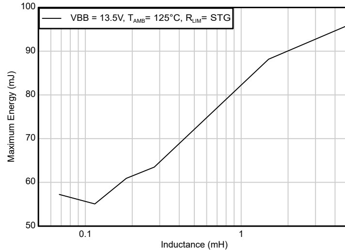
図 8-28. 誘導性スイッチ オフ時の最大エネルギー吸収量 対 インダクタンス (シングルパルス、VBB = 13.5V、TA = 125°C)
