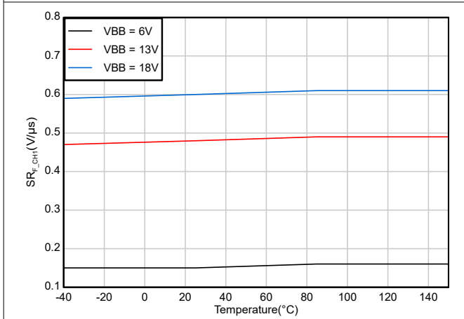
図 6-15. VOUT 下降スルー レート (SR F ) 対 温度 (チャンネル 1 : P パッケージ)
