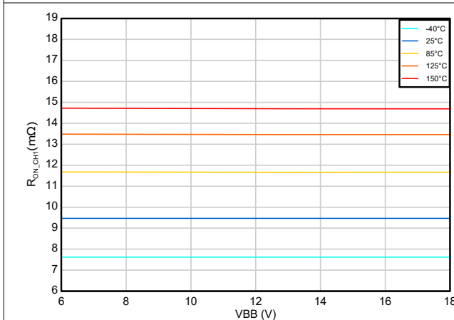
図 6-5. オン抵抗 ( R_{ON} ) 対 VBB 特性 (チャンネル 1)
