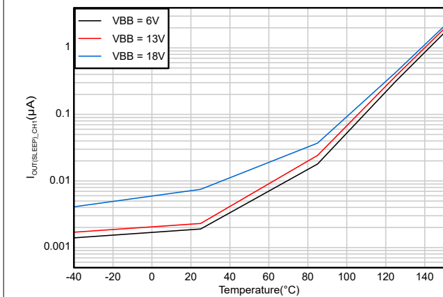
図 6-3. 出力リーク電流 ( I_{OUT(SLEEP)} ) 対温度特性 (チャンネル 1)
