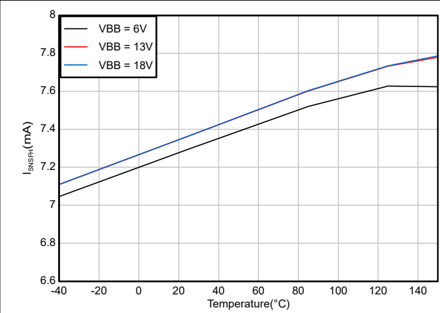
図 6-8. I_{SNS} フォルト 高レベル電流 対 温度
