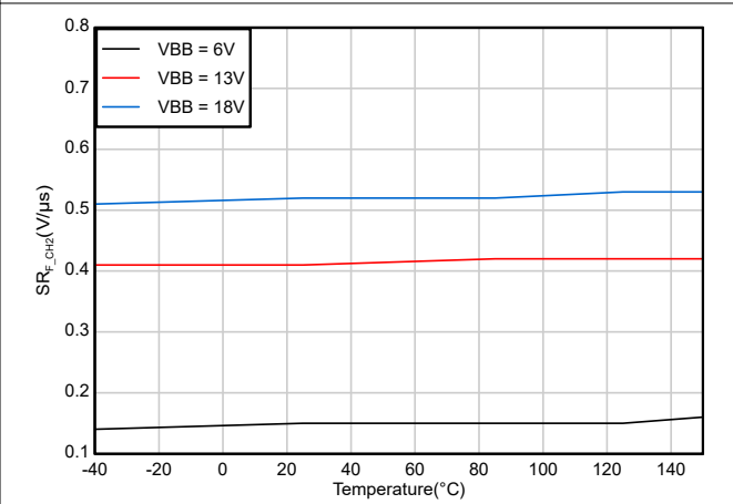
図 6-16. VOUT 下降スルー レート (SR F ) 対 温度 (チャンネル 2 : P パッケージ)
