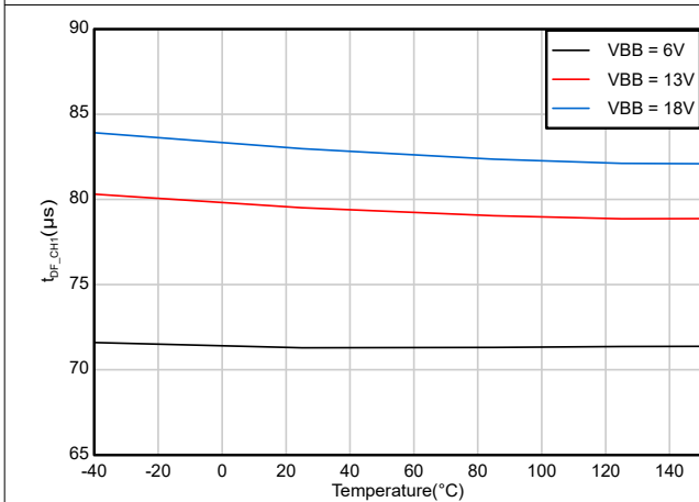
図 6-11. チャネル ターンオフ遅延時間 ( t_{DF} ) 対 温度 (チャネル 1)
