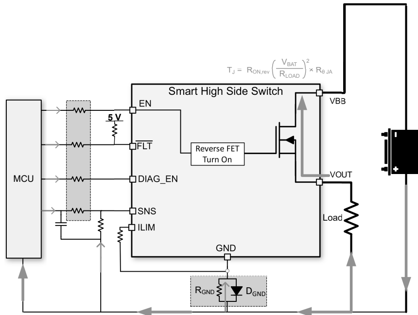
図 8-44. GND ネットワークによるリバーブ プロテクション
