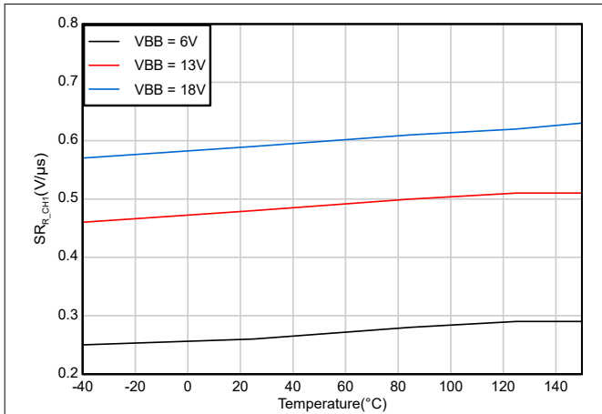
図 6-13. VOUT 上昇スルー レート (SR R ) 対 温度 (チャンネル 1 : P パッケージ)
