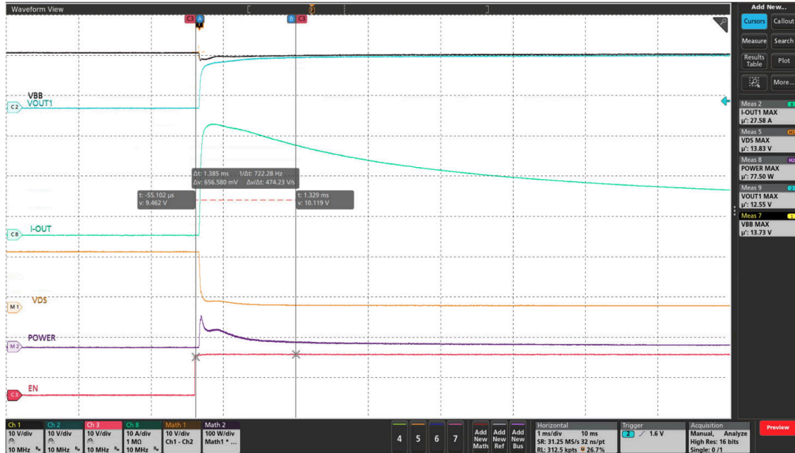
図 8-35. 13.5V VBB 条件下における TPS2HC08-Q1 シングル チャネル使用時の 35W 電球 充電特性、 T_A (device) = 25°C、 T_A (bulb) = 25°C、ILIM = GND
