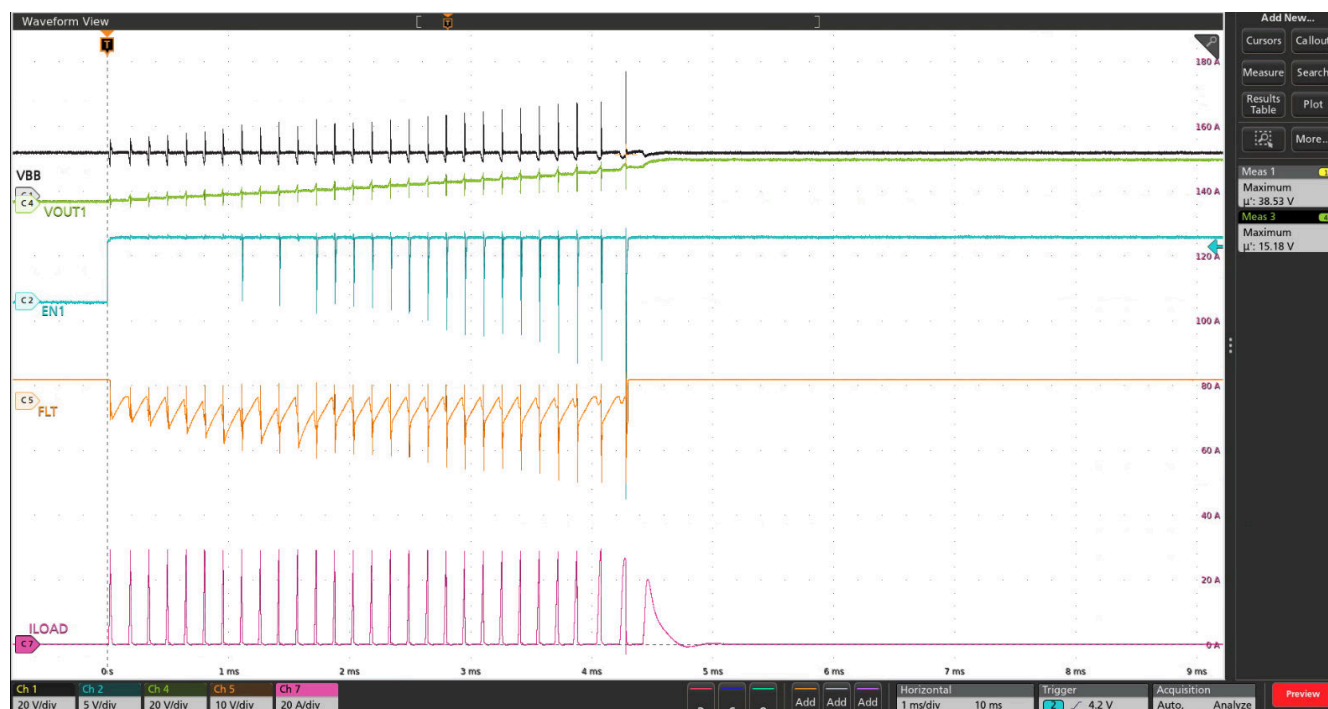
図 8-30. 13.5V の VBB、ILIM ピン短絡 (GND 接続)、周囲温度 125°C、かつチャンネル 2 に負荷なしという条件における、TPS2HC08-Q1 デバイスのチャンネル 1 による 1mF 容量性負荷の充電。
