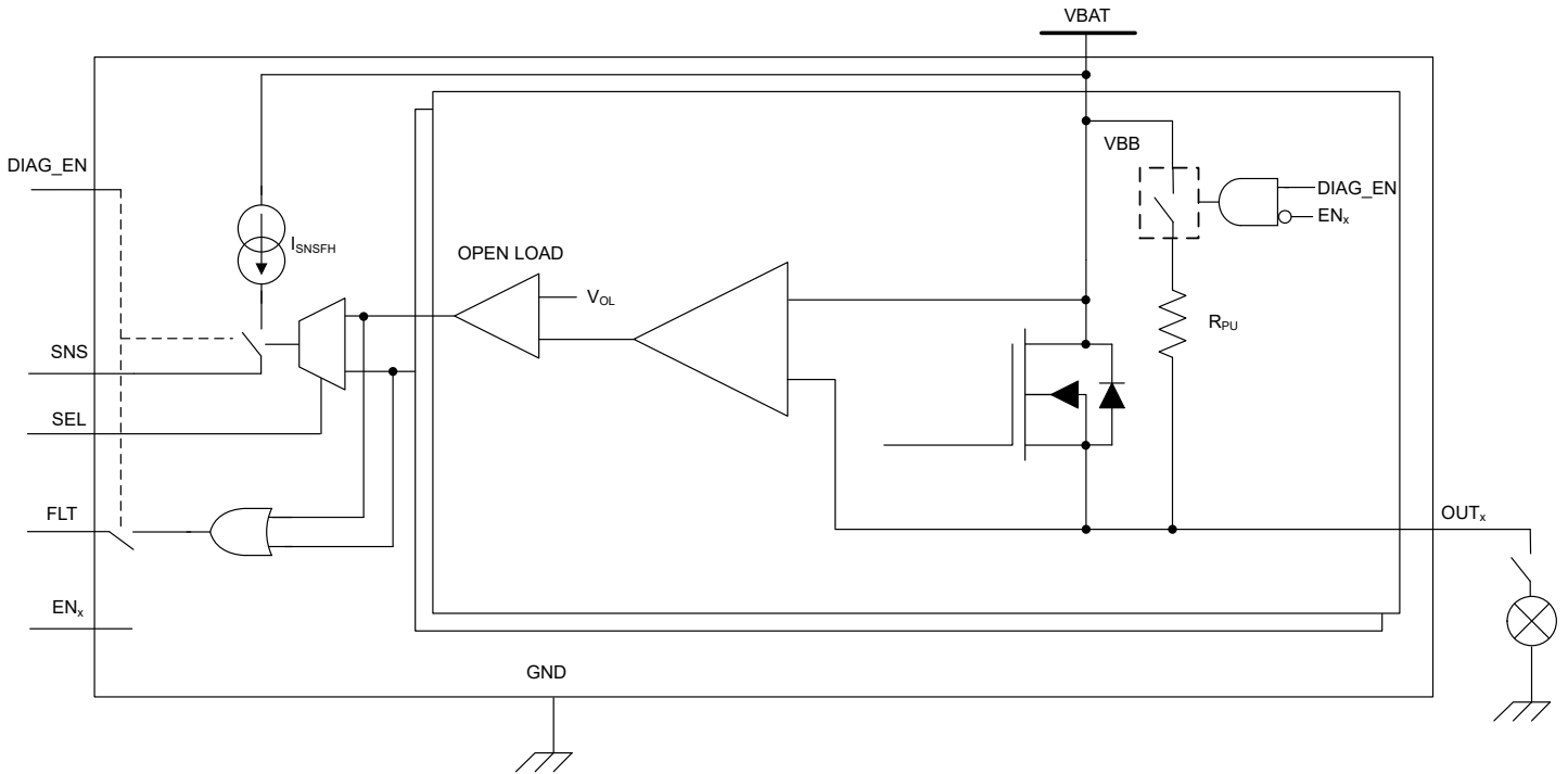
図 8-37. オフ状態での開放負荷検出
