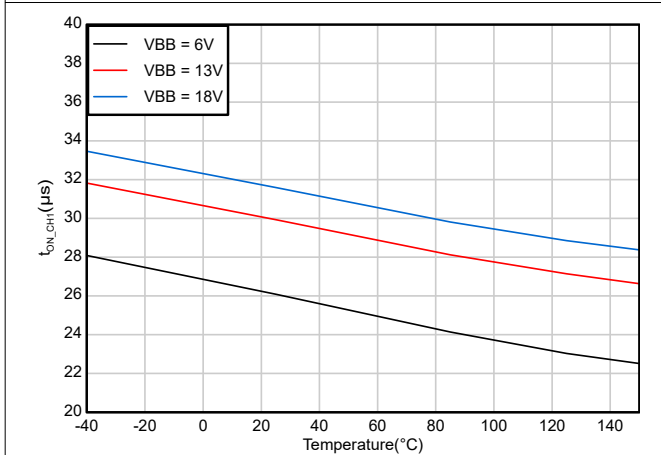
図 6-17. チャンネル ターンオン時間 (t ON ) 対 温度 (チャンネル 1)
