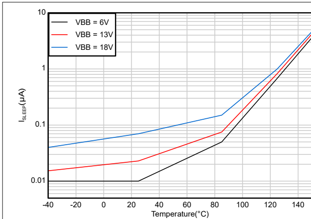
図 6-1. スタンバイ電流 ( I_{SLEEP} ) 対温度
