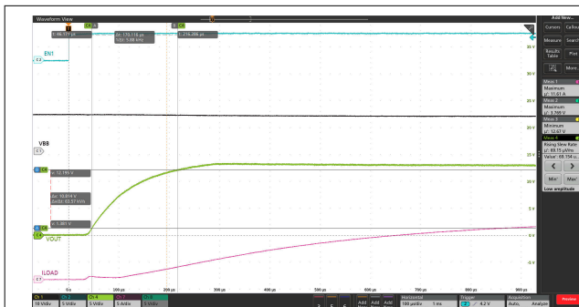
図 9-3. 抵抗性負荷でのターンオン
