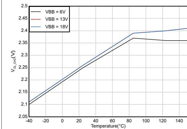
図 6-27. 開放負荷の検出 電圧 (V OL ) 対 温度 (チャネル 2)
