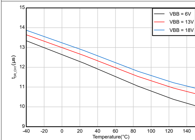
図 6-9. チャネル ターンオン遅延時間 ( t_{DR\_CH1} ) 対 温度 (チャネル 1)
