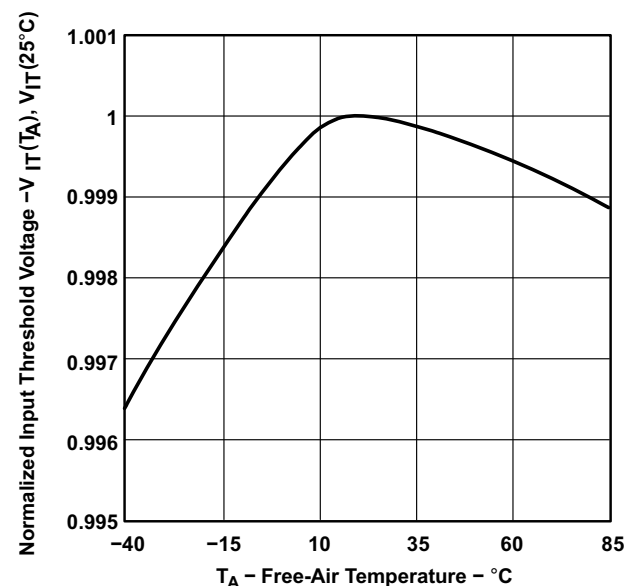
正規化された入力スレッショルド電圧と自由通気温度との関係
