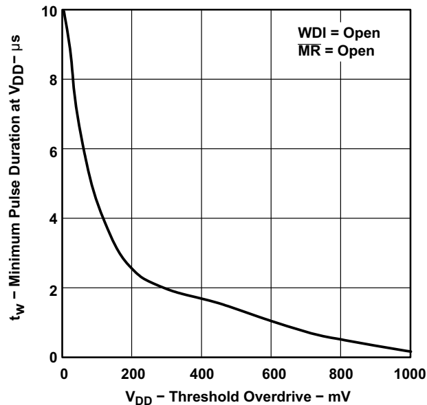
図 8-2. V DD の最小パルス幅と V DD スレッシュホルド・オーバードライブとの関係
