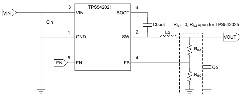
TPS54202x の概略回路図
