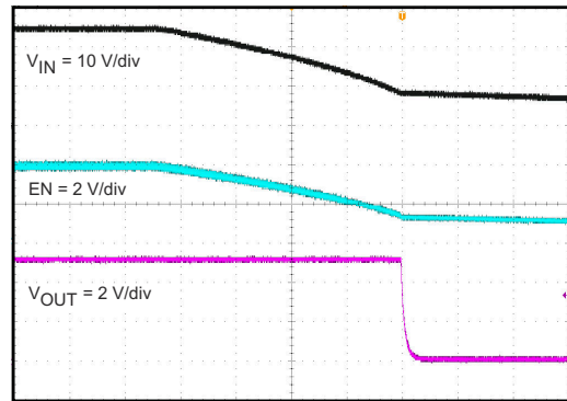
图 8-11. Transient Response
