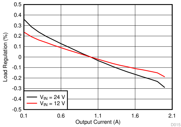
图 8-4. Load Regulation
