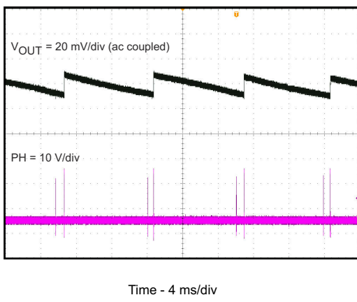
图 8-6. Output Voltage Ripple
