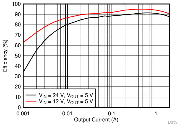
图 8-2. Efficiency
