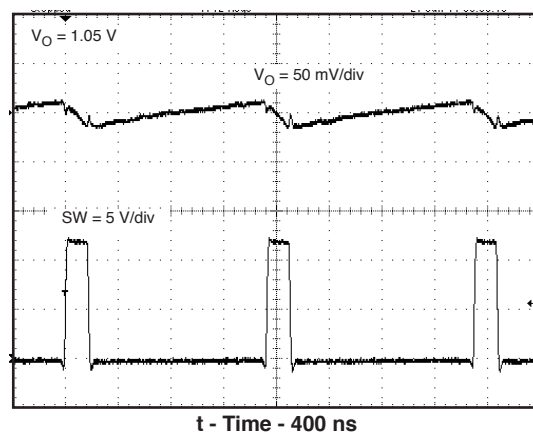
図 12. 入力電圧リップル (I O = 2A)
