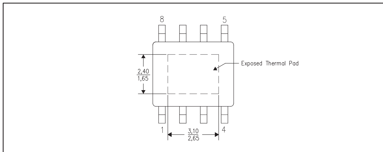
図 15. サーマル・パッドの寸法(平面図)
