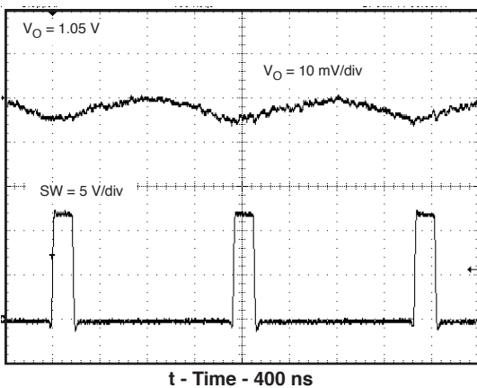
図 11. 出力電圧リップル (I O = 2A)
