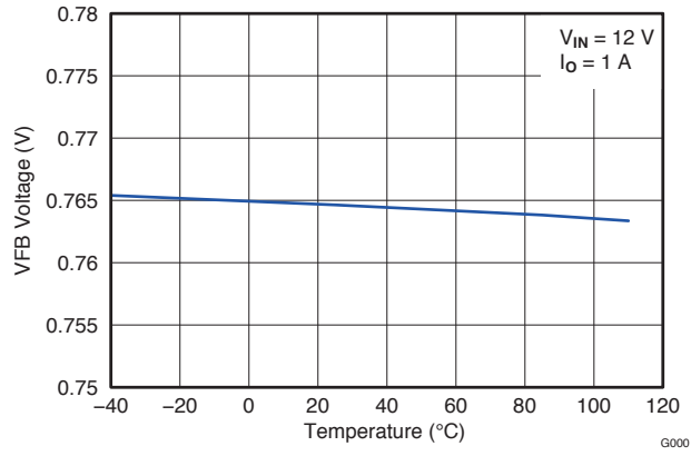
図 13. VFB電圧 对 接合部温度
