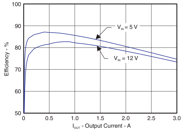
図 8. 効率 対 出力電流
