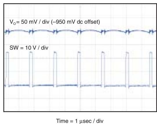
図 12. 出力電圧リップル (I O = 3A)
