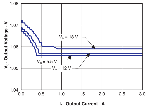
図 4. 1.05V出力電圧 対 出力電流
