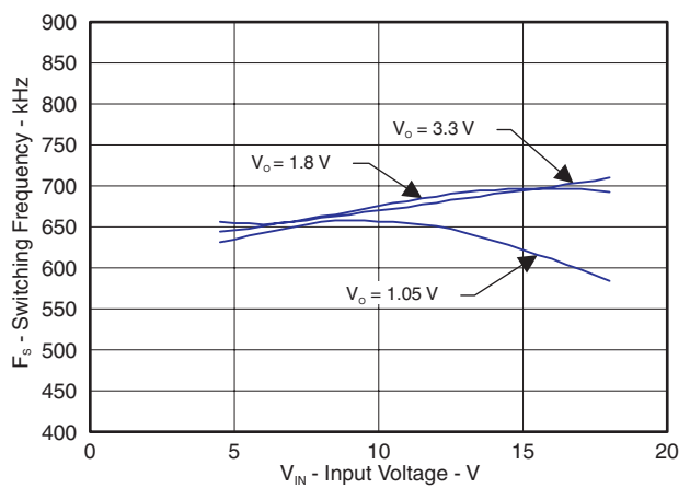
図 10. スイッチング周波数 対 入力電圧
