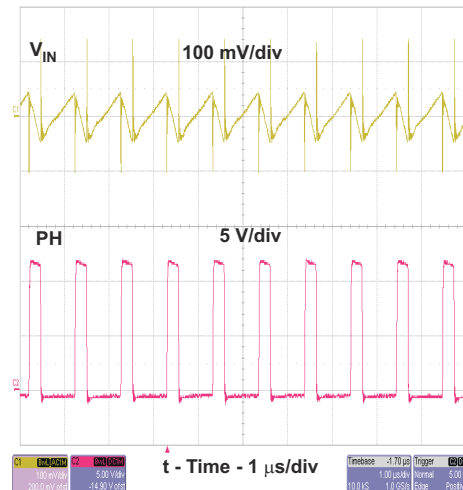
図 8-9. TPS54332 Input Ripple
