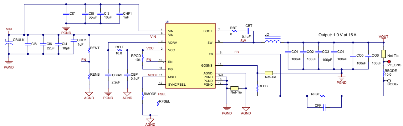
図 7-1. 12V Input, 1.0V Output, 1MHz Schematic
