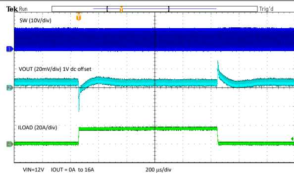
図 7-8. Load Transient
