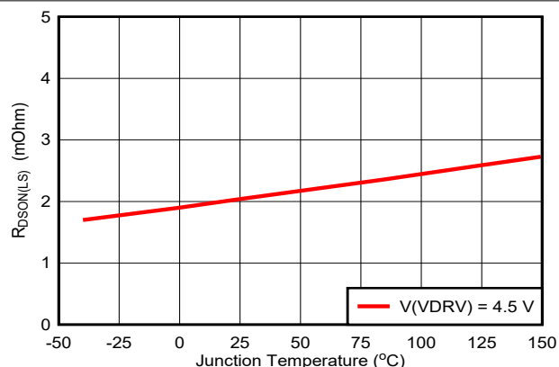
図 5-2. Low-Side FET R_{DS(on)}
