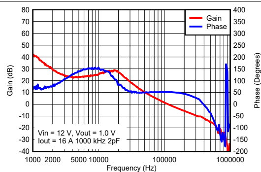
図 7-7. Bode Plot
