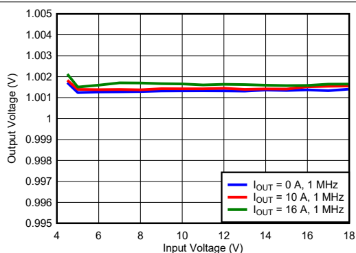
図 7-6. Line Regulation
