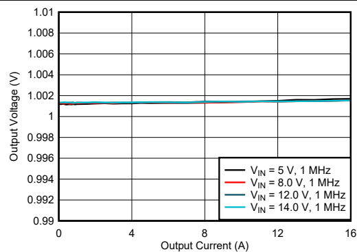
図 7-5. Load Regulation
