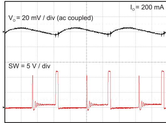
图 25. TPS562210A Output Voltage Ripple
