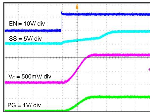
图 29. TPS562210A Start Up Relative To En
