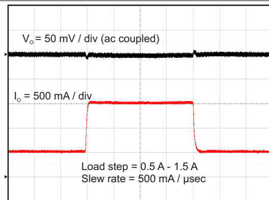
图 27. TPS562210A Transient Response
