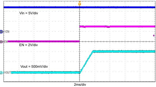
図 7-15. EN によるスタートアップ、 I_{OUT} = 3A
