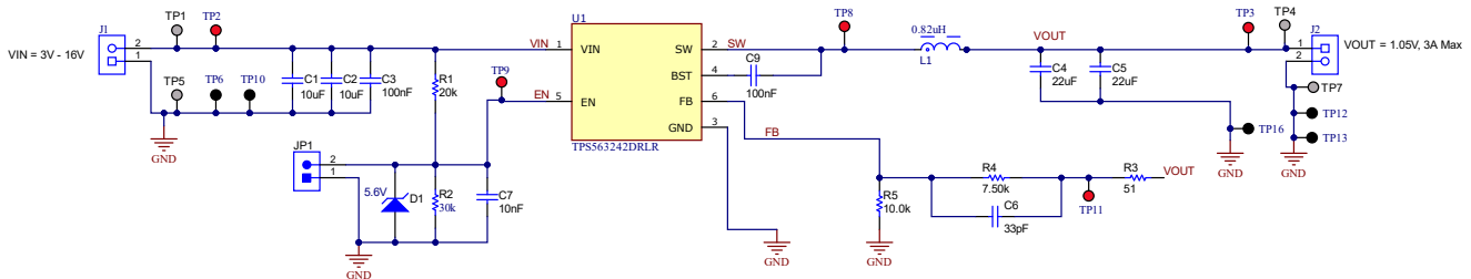
図 7-1. 回路図
