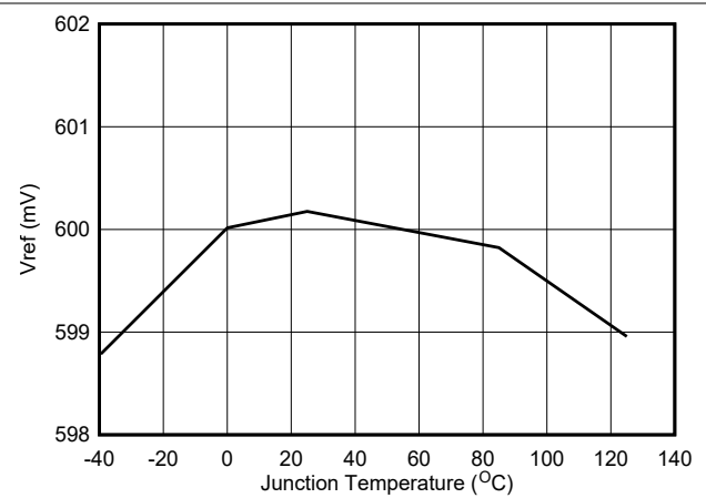
图 5-2. V_{ref} Voltage
