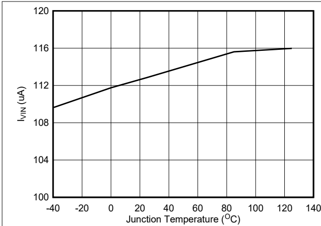
图 5-1. TPS563203 Quiescent Current
