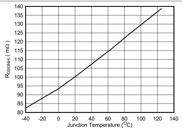
图 5-6. High-Side R_{dson}
