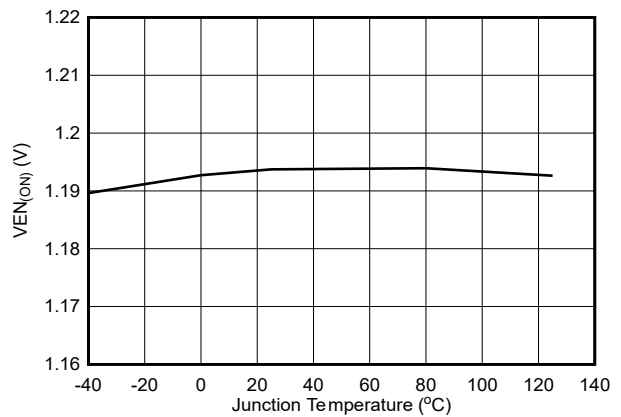
図 5-4. イネーブル オン スレッシュホールド電圧
