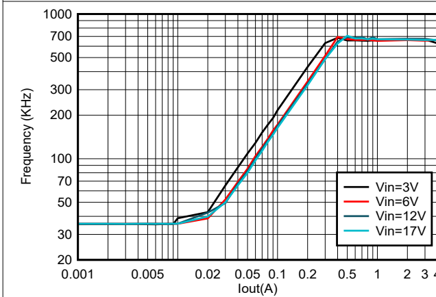
図 7-4. TPS564255B 周波数と負荷との関係
