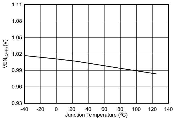
図 5-5. イネーブル オフ スレッシュホールド電圧
