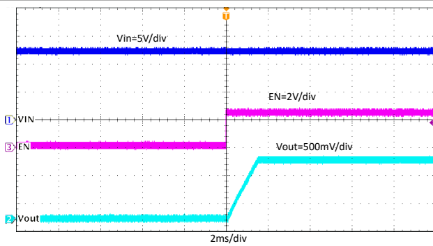
図 7-18. EN によるスタートアップ、 I_{OUT} = 4A
