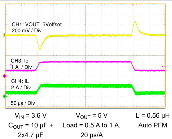
9-7. Load Transient
