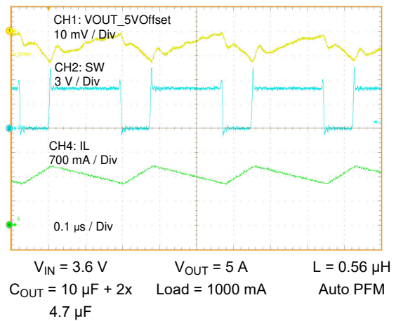
9-3. Steady 1000 mA
