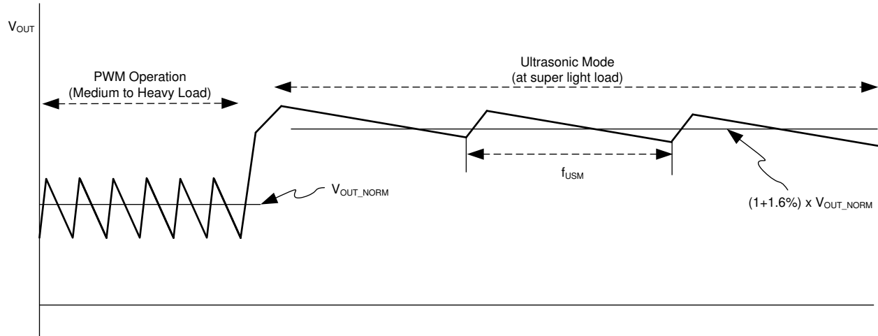
図 8-4. Ultrasonic Mode Operation
