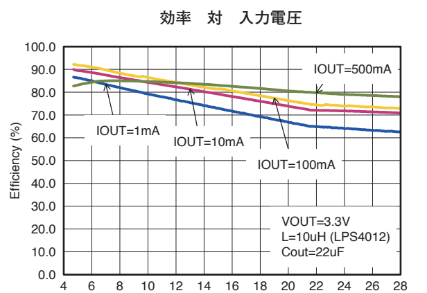
図 10. Vout = 3.3V
