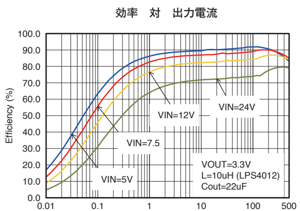
図 9. Vout = 3.3V
