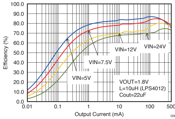
図 13. Vout = 1.8V
