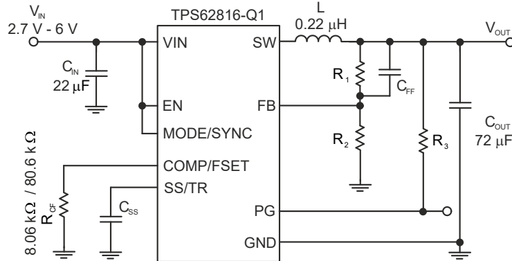
图 10-62. Schematic
