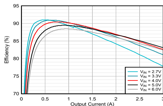
降圧コンバータの効率と I_{OUT} との関係 ( V_{OUT} = 1.1\text{V} )
