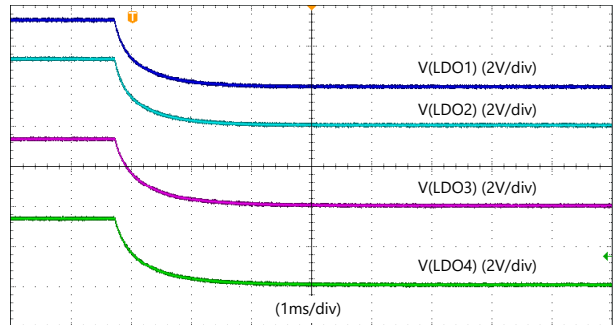
7-9. LDOs Discharge
