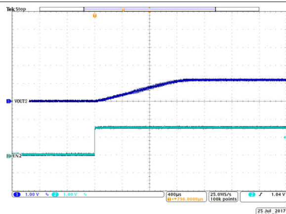
图 8-4. BUCK2 Soft-Start
