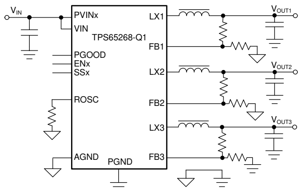
アプリケーション回路図
