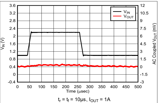
図 5-20. ライン過渡変化 : 1V ~ 2.2V
