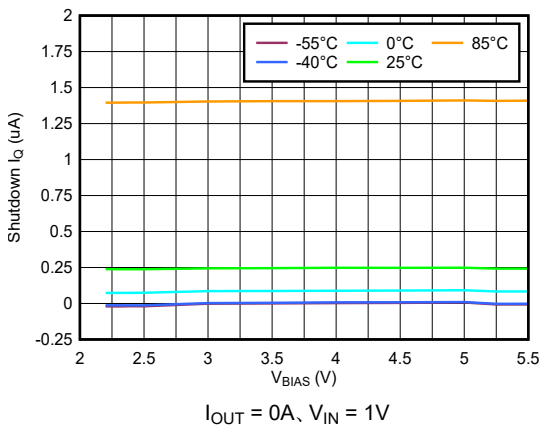
図 5-9. V_{\text{BIAS}} シャットダウン I_Q と V_{\text{BIAS}} との関係 I_{\text{OUT}} = 0\text{A} 、 V_{\text{IN}} = 1\text{V}
