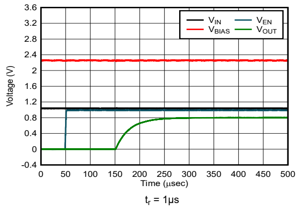
図 5-16. V_{\text{IN}} および V_{\text{BIAS}} が V_{\text{EN}} より先に印加された場合の起動
