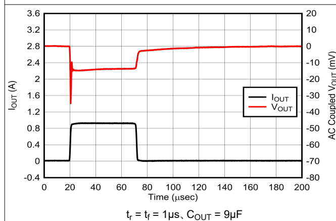
図 5-21. 負荷過渡応答 : 100µA ~ 1A
