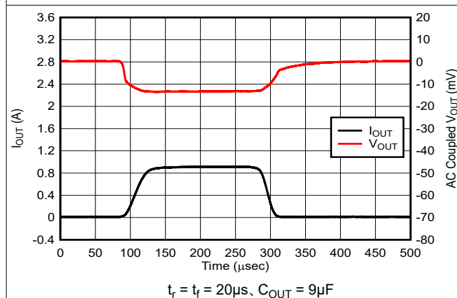
図 5-23. 負荷過渡応答 : 100µA ~ 1A
