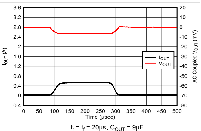
図 5-24. 負荷過渡応答 : 10mA ~ 500A
