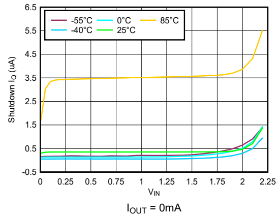
図 5-8. V_{\text{IN}} シャットダウン I_Q と V_{\text{IN}} との関係 I_{\text{OUT}} = 0\text{mA}
