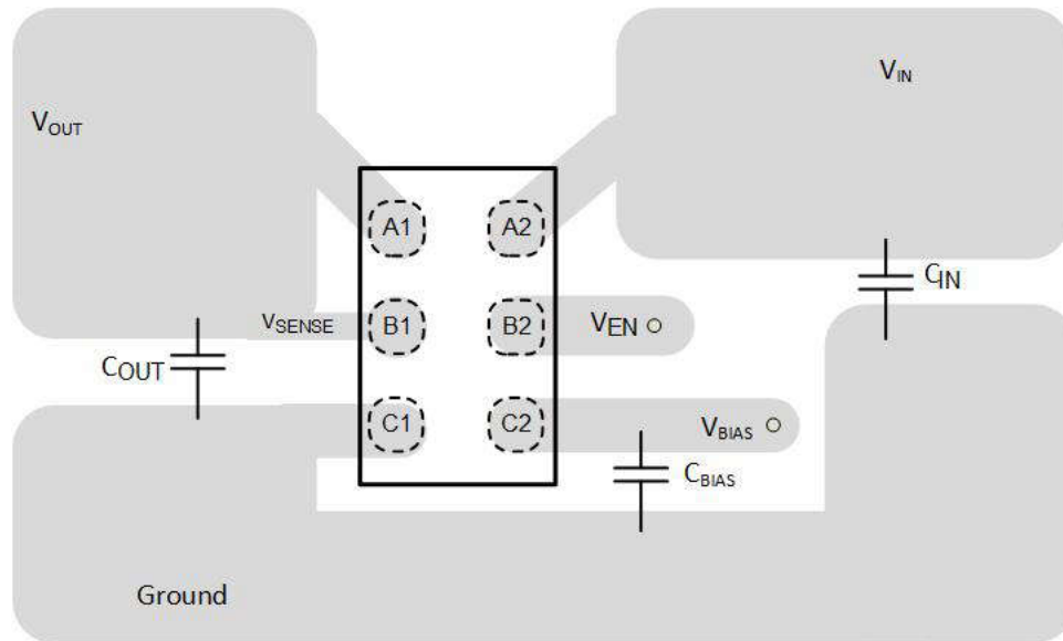
図 7-6. 推奨レイアウト (YBK パッケージ)
