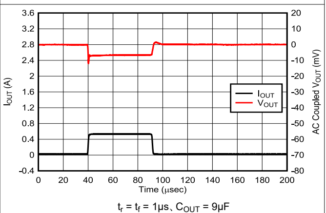
図 5-22. 負荷過渡応答 : 10mA ~ 500mA
