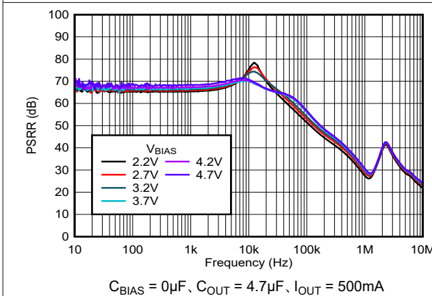
図 5-29. V_{BIAS} - V_{OUT} における PSRR と周波数との関係
