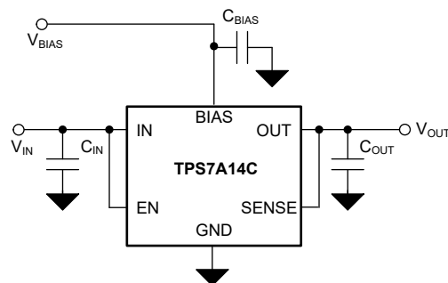
代表的なアプリケーション回路
