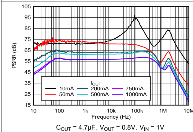
図 5-27. PSRR と周波数および I_{OUT} との関係
