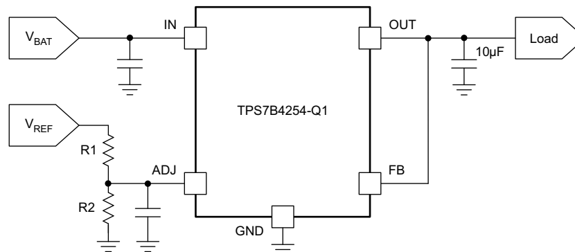
図 6-5. 基準電圧より低い OUT 電圧
