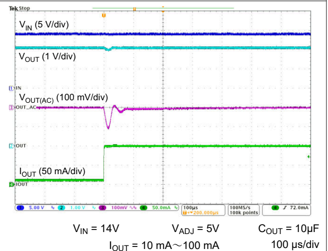
図 5-20. 10V から 100mA への負荷過渡
