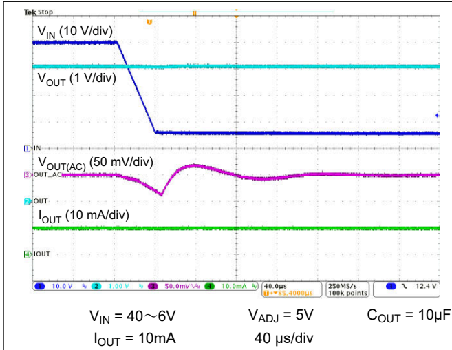
図 5-17. 40V ~ 6V へのライン過渡
