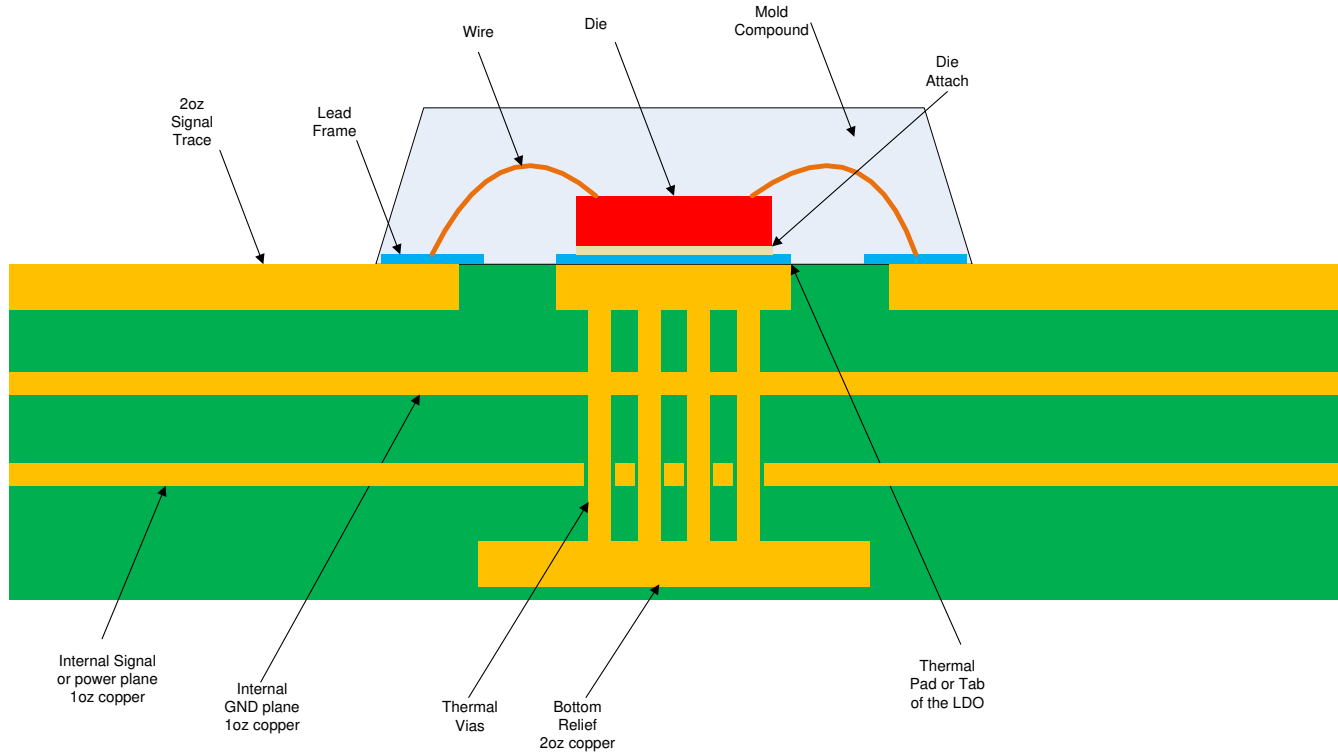
☒ 7-8. JEDEC Standard 2s2p PCB
