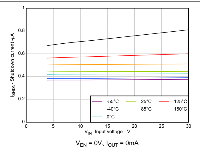
図 5-14. シャットダウン電流と入力電圧との関係
