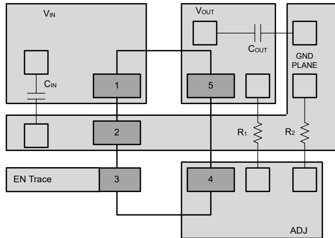
図 7-11. TPS7E71、DBV パッケージのレイアウト例
