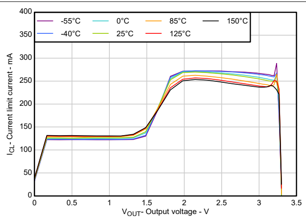
図 5-10. 電流制限と出力電圧との関係
