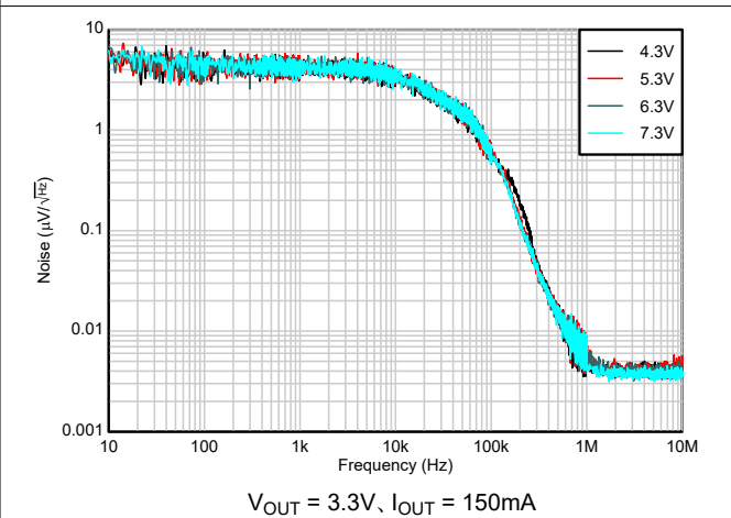
図 5-24. 出力ノイズと周波数、入力電圧との関係
