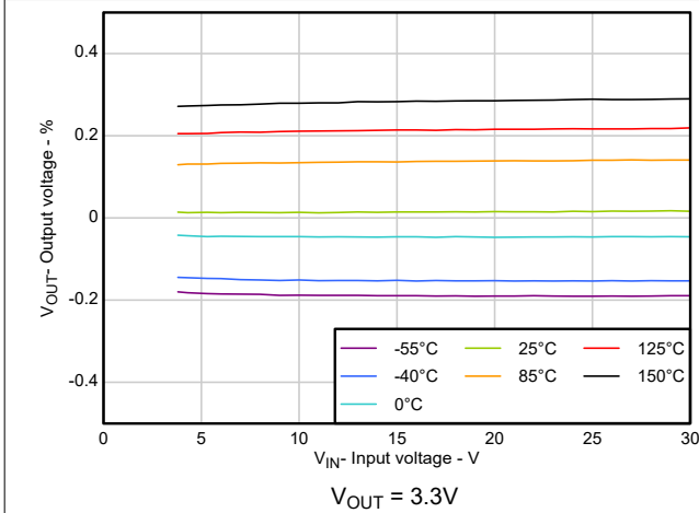
図 5-3. 精度と入力電圧との関係
