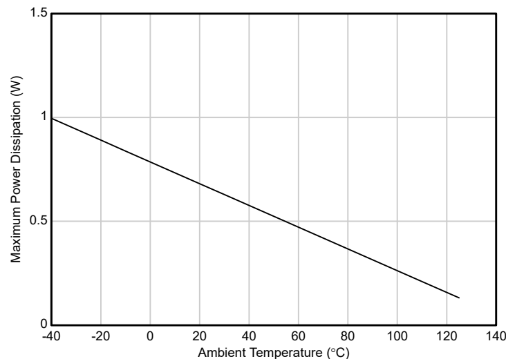
図 7-2. TPS7E71 (DBV) 許容消費電力
