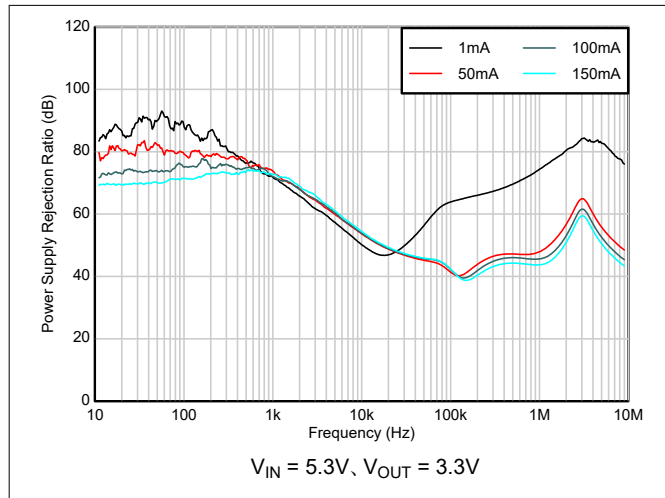
図 5-21. リップル除去と周波数、出力電流との関係
