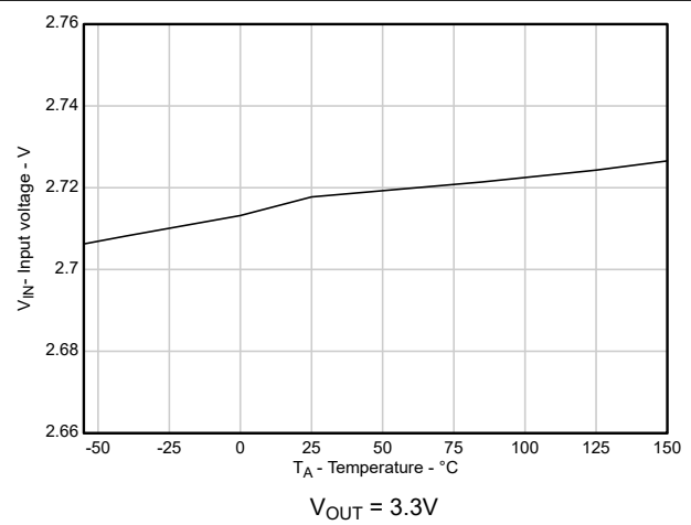
図 5-2. 立ち下がり入力電源 UVLO と温度との関係
