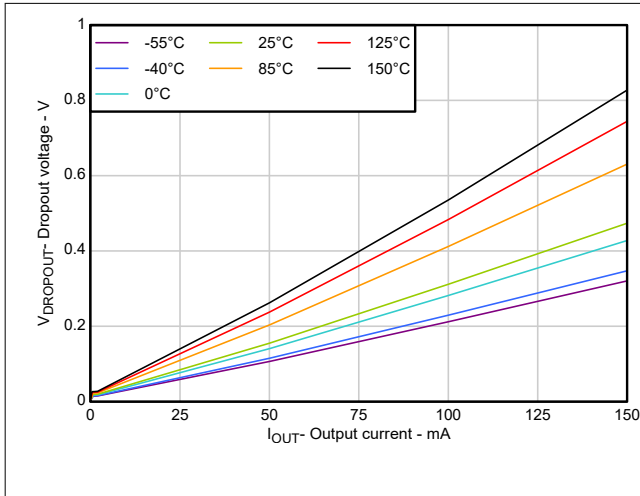
図 5-9. ドロップアウトと出力電流との関係
