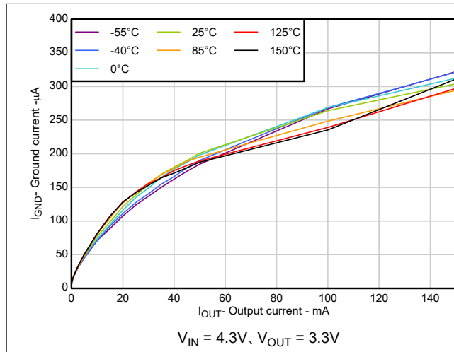
図 5-13. グランド電流と出力電流との関係
