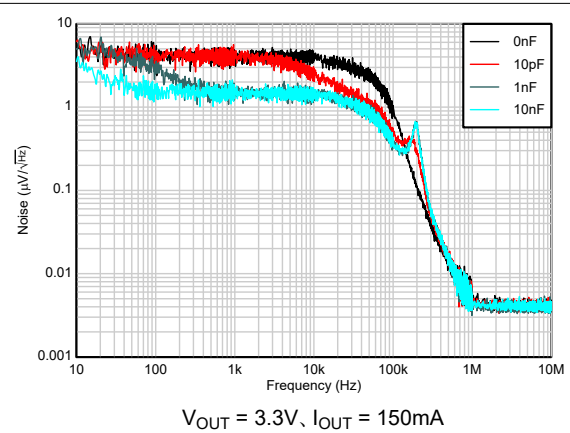
図 5-26. 出力ノイズ密度と周波数および C_{FF} との関係
