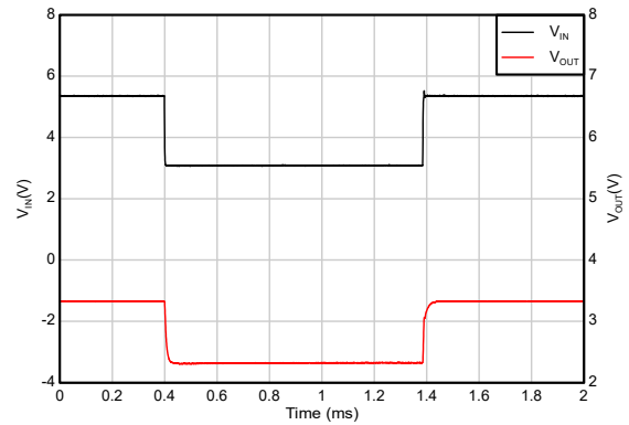
V_{IN} = 5.3\text{V} \sim 3\text{V} 、 V_{OUT} = 3.3\text{V} 、 I_{OUT} = 300\text{mA} 、スルーレート = 2\text{V}/\mu\text{s}
