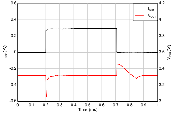
I_{OUT} = 0\text{mA} \sim 300\text{mA} 、 V_{IN} = 5.3\text{V} 、 V_{OUT} = 3.3\text{V} 、スルーレート = 2\text{A}/\mu\text{s}
