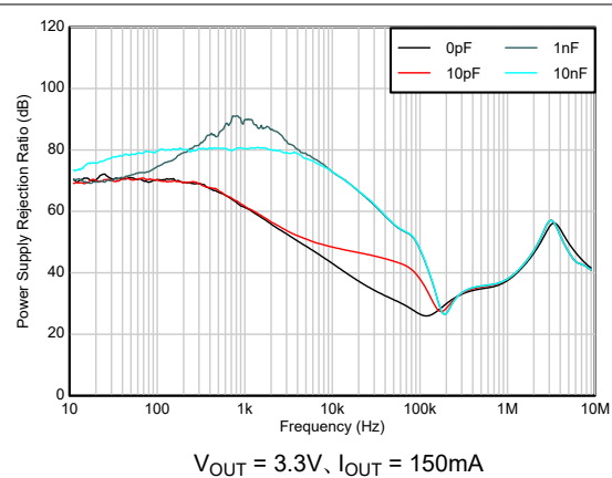
図 5-22. リプル除去と周波数、 C_{FF} との関係
