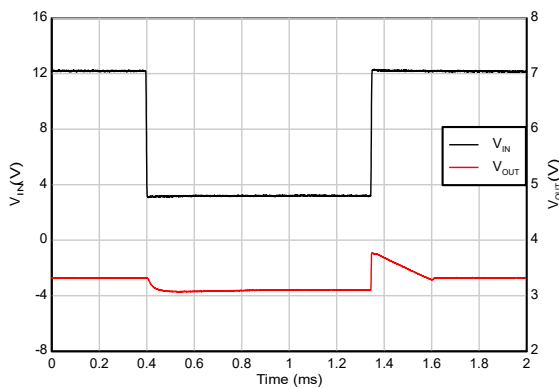
V_{IN} = 12\text{V} \sim 3\text{V} 、 V_{OUT} = 3.3\text{V} 、スルーレート = 2\text{V}/\mu\text{s}
