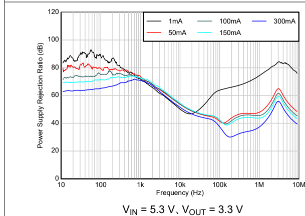
図 5-21. リプル除去と周波数、出力電流との関係
