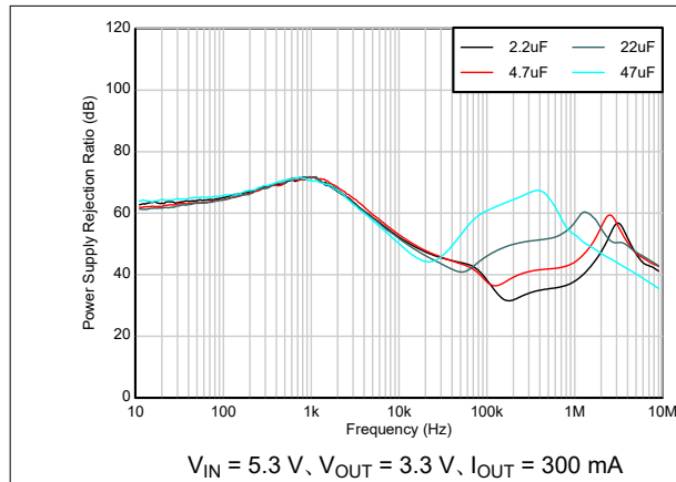
図 5-19. リプル除去と周波数、 C_{OUT} との関係
