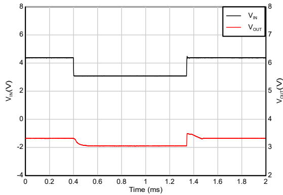
V_{IN} = 4.3\text{V} \sim 3\text{V} 、 V_{OUT} = 3.3\text{V} 、スルーレート = 2\text{V}/\mu\text{s}
