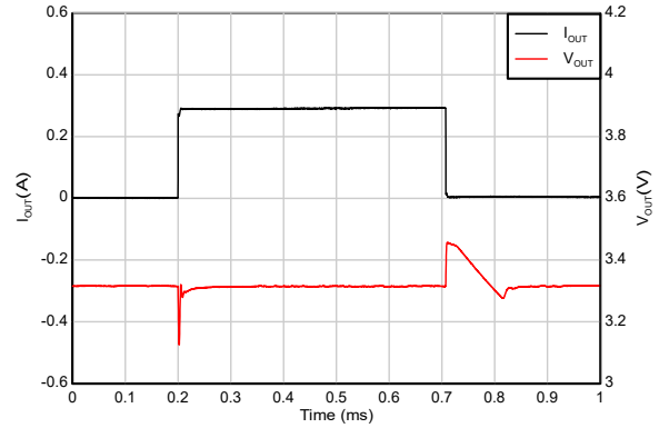
I_{OUT} = 1\text{mA} \sim 300\text{mA} 、 V_{IN} = 5.3\text{V} 、 V_{OUT} = 3.3\text{V} 、スルーレート = 2\text{A}/\mu\text{s}
