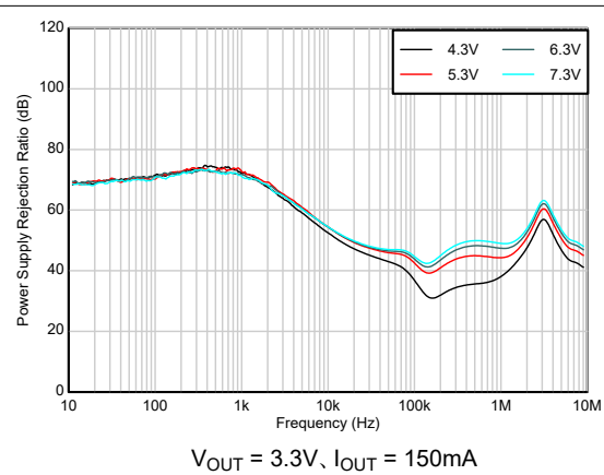
図 5-20. リプル除去と周波数、入力電圧との関係
