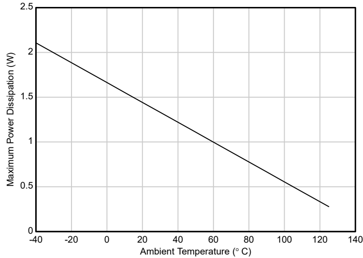
図 7-3. TPS7E72 (DRV) 許容消費電力
