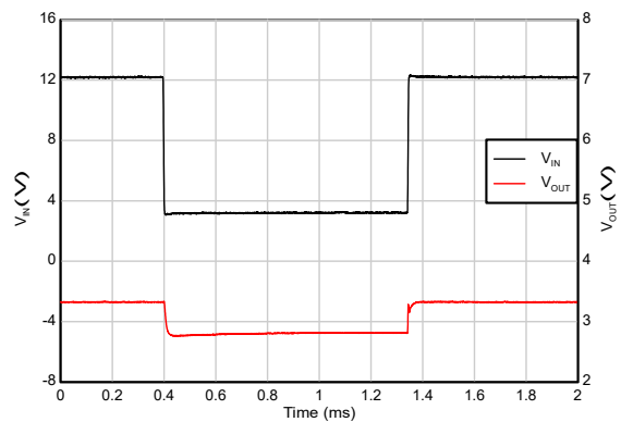
V_{IN} = 12\text{V} \sim 3\text{V} 、 V_{OUT} = 3.3\text{V} 、 I_{OUT} = 100\text{mA} 、スルーレート = 2\text{V}/\mu\text{s}
