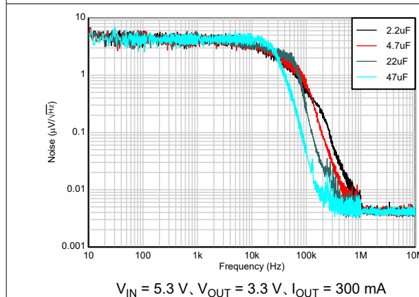
図 5-23. 出力ノイズ密度と周波数および C_{OUT} との関係
