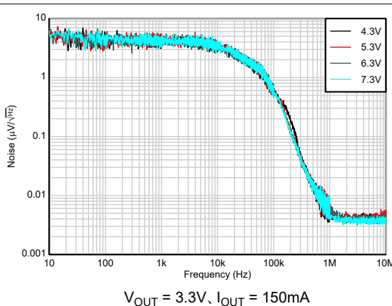
図 5-24. 出力ノイズと周波数、入力電圧との関係
