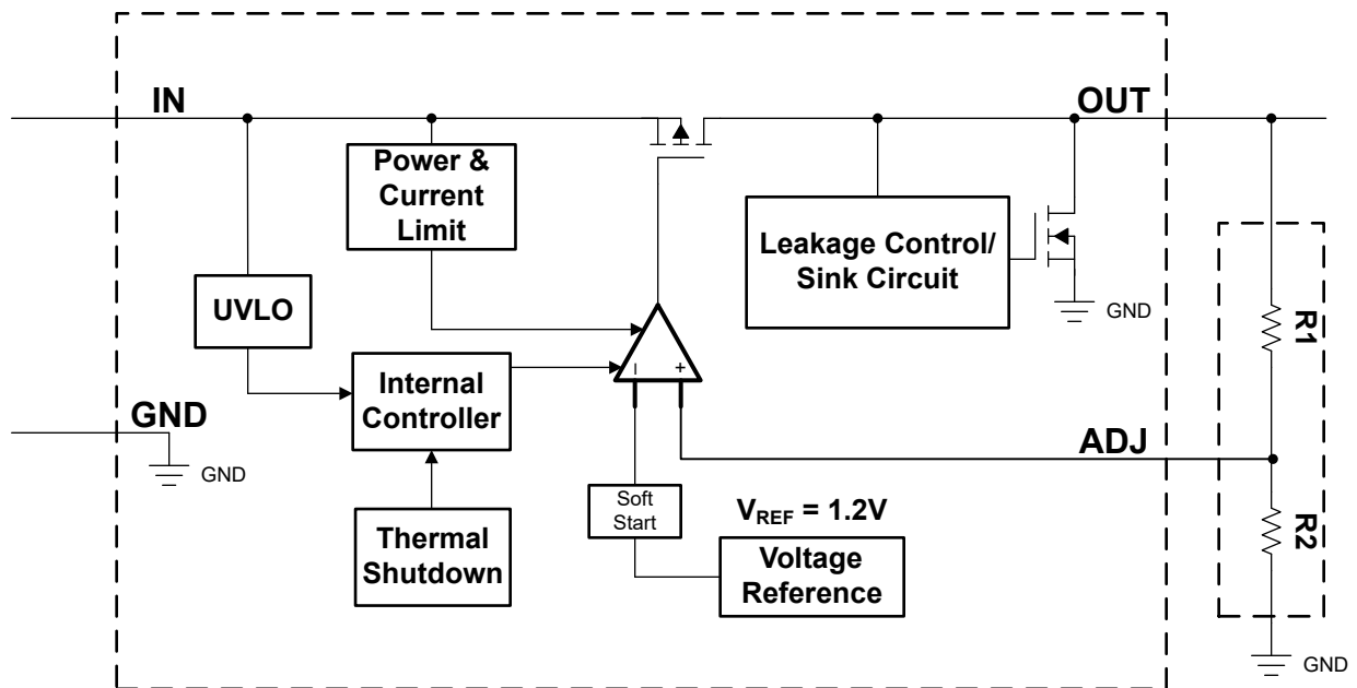
図 6-3. 機能ブロック図：可変バージョン (EN 機能なし)
