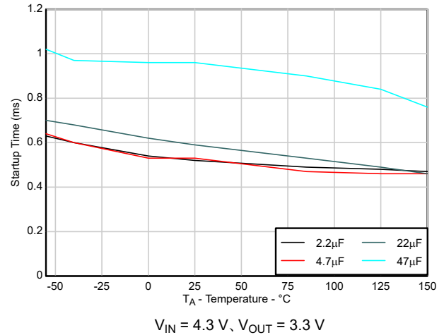
図 5-18. スタートアップタイムと C_{\text{OUT}} との関係
