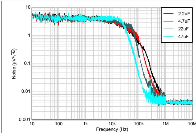
図 5-25. ノイズと C_{OUT} との関係
