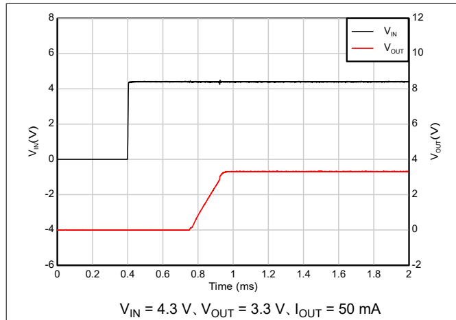
図 5-31. EN & V_{IN} を互いに接続した状態でのスタートアップ
