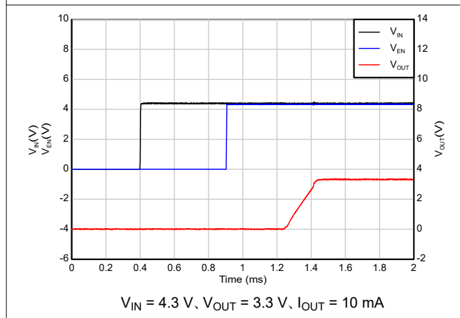
図 5-33. シーケンスによる起動 ( V_{IN} 後の EN)
