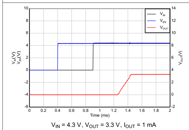
図 5-35. シーケンスによる起動 (EN 後ろの V_{IN} )
