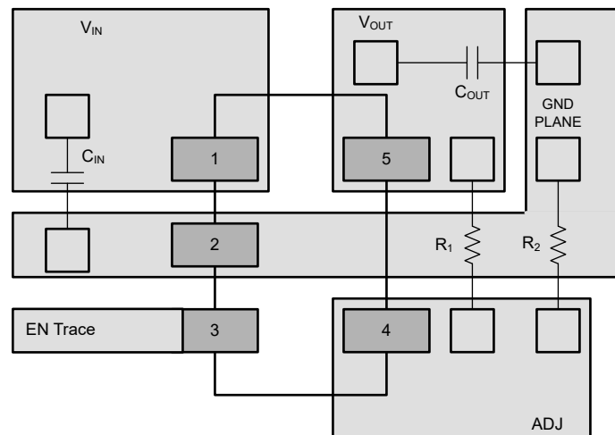
図 7-20. DBV パッケージのレイアウト例
