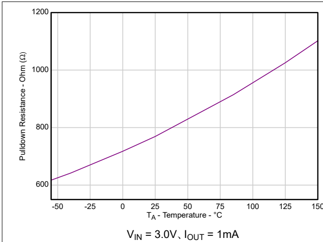
図 5-17. 出力のプルダウン抵抗 ( R_{\text{Discharge}} ) と温度との関係
