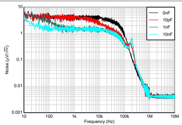
図 5-26. ノイズと C_{FF} との関係
