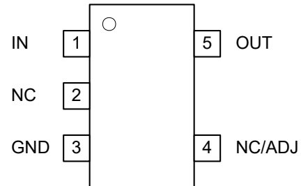
図 4-4. DBV パッケージ、[A バージョン、EN なし] (固定/可変)、5 ピン SOT-23 (上面図)
