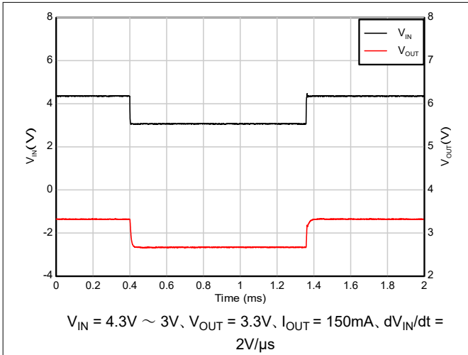
図 5-45. ドロップアウトからの回復 (4.3V 入力 3V 出力)
