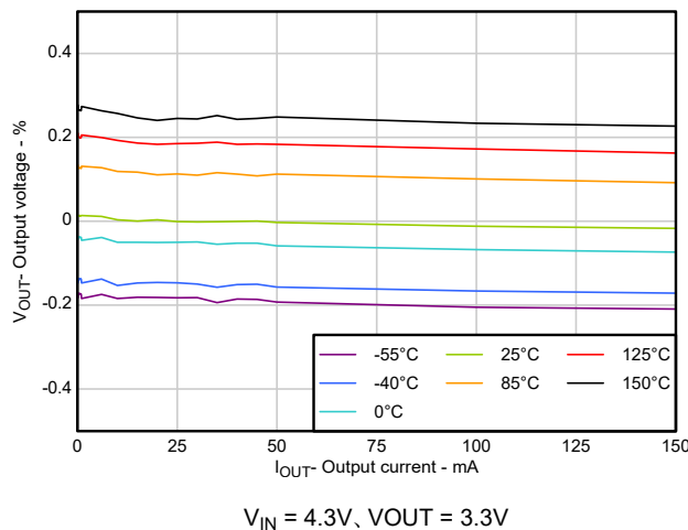
図 2-1. V_{\text{OUT}} の精度と I_{\text{OUT}} との関係
