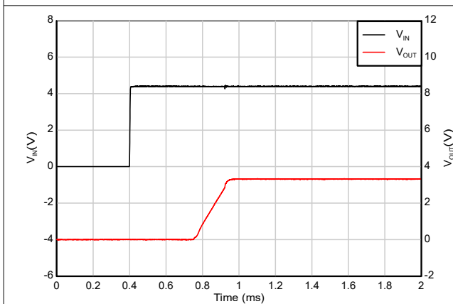
図 5-27. スタートアップと C_{OUT} との関係
