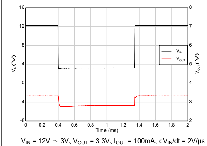
図 5-47. ドロップアウトからの回復 (12V 入力 3V 出力)
