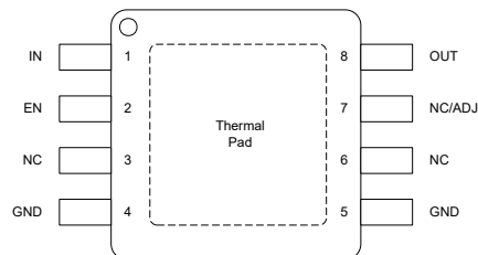
図 4-5. DGN パッケージ (固定/可変)、8 ピン HVSSOP (上面図)
