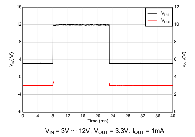
図 5-48. コールドクランク回復
