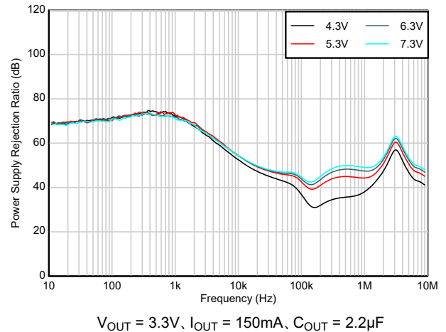
図 5-20. PSRR と V_{IN} との関係
