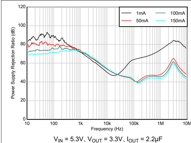
図 5-19. PSRR と I_{\text{OUT}} との関係
