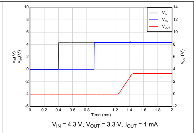
図 5-32. シーケンスによる起動 ( V_{IN} 後の EN)
