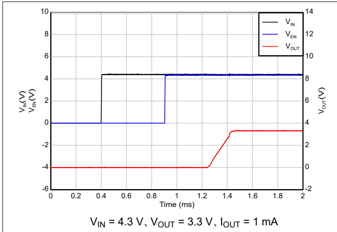
図 5-31. シーケンスによる起動 ( V_{IN} 後の EN)
