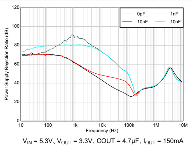
図 5-22. PSRR と C_{FF} との関係
