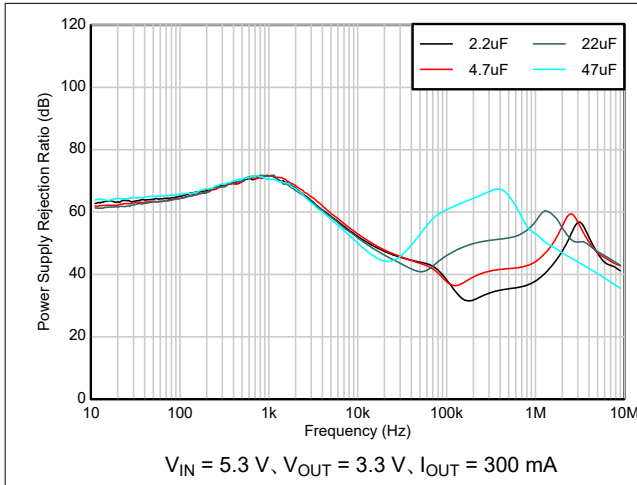
図 5-21. PSRR と C_{OUT} との関係
