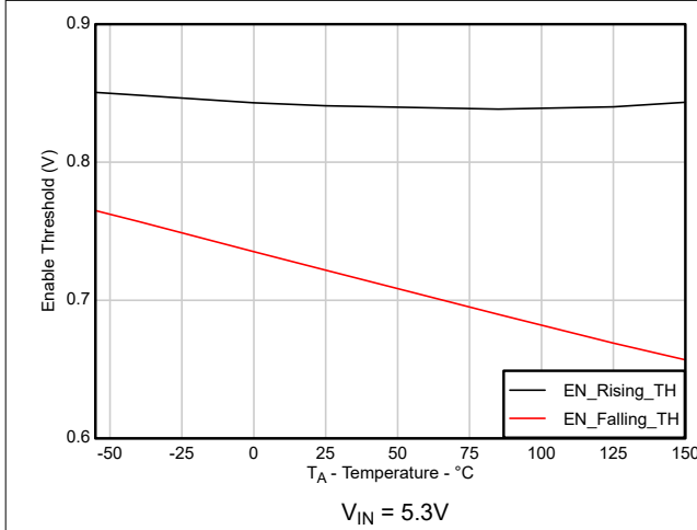
図 5-13. EN スレッシュヨルド V_{IH(EN)}/V_{IL(EN)} と温度との関係
