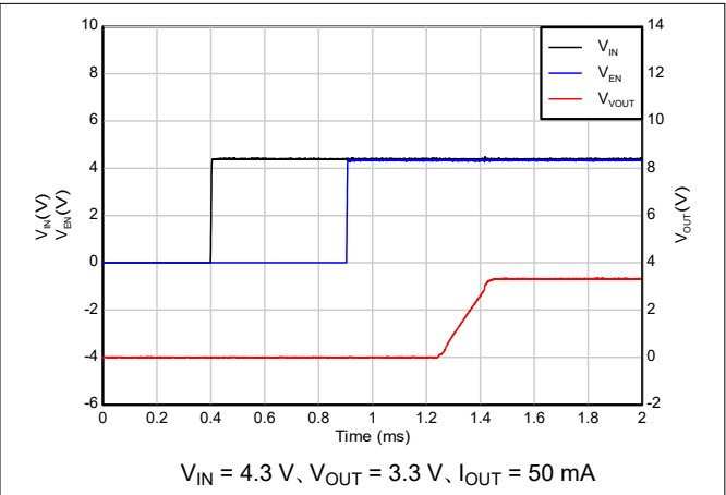
図 5-32. シーケンスによる起動 ( V_{IN} 後の EN)
