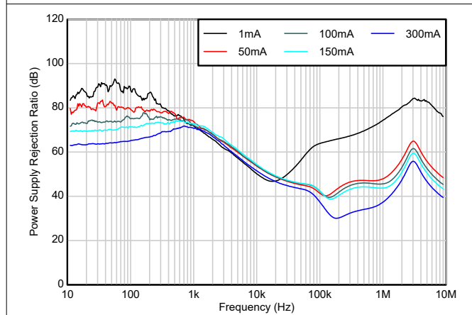
図 5-19. PSRR と I_{OUT} との関係
