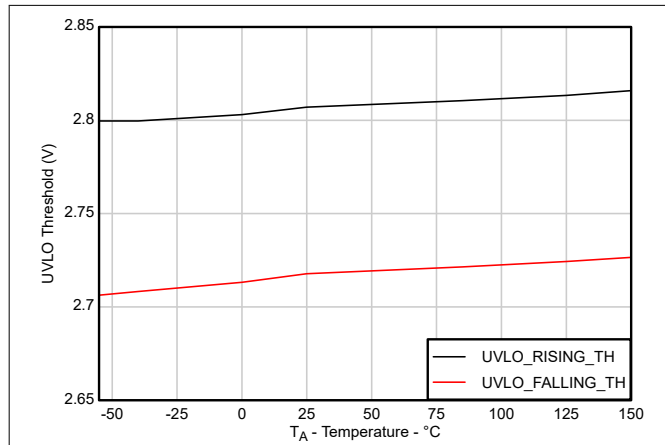
図 5-17. UVLO スレッシュホールド ( V_{UVLO+}/V_{UVLO-} ) と温度との関係
