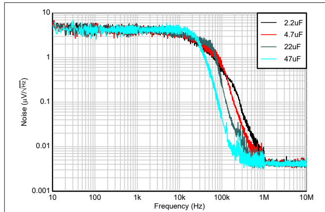
図 5-25. ノイズと C_{OUT} との関係
