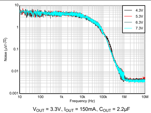
図 5-24. ノイズと V_{IN} との関係
