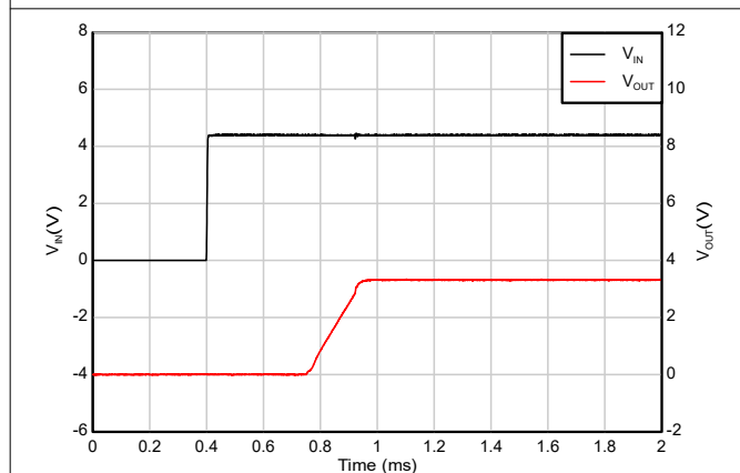
図 5-27. スタートアップと C_{OUT} との関係
