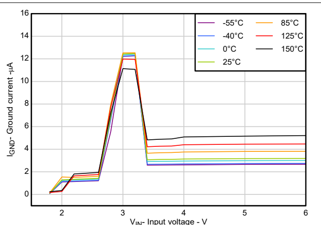
図 5-8. I_{GND} と V_{IN} との関係
