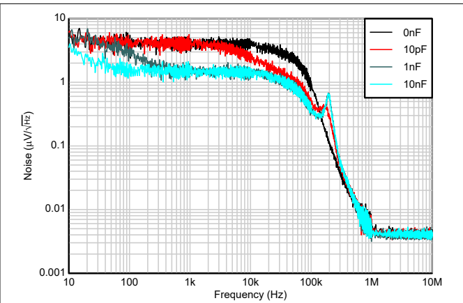
図 5-26. ノイズと C_{FF} との関係
