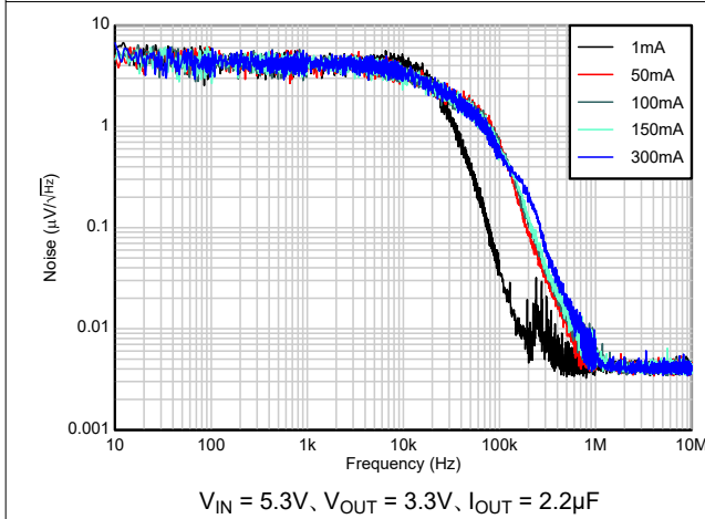
図 5-23. ノイズと I_{OUT} との関係
