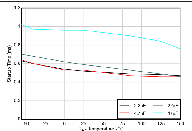
図 5-18. スタートアップタイムと C_{OUT} との関係
