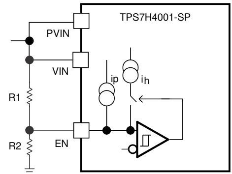
8-3. Adjustable VIN and PVIN UVLO
